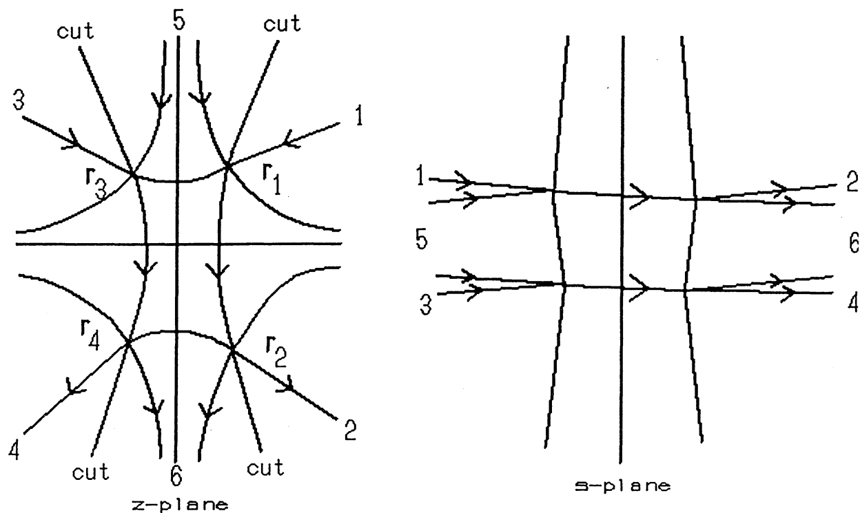
図2 z -平面と s -平面の状況
