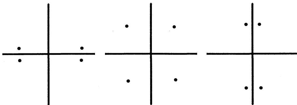
図 1 原子衝突過程の解析で現れる転回点の状況
