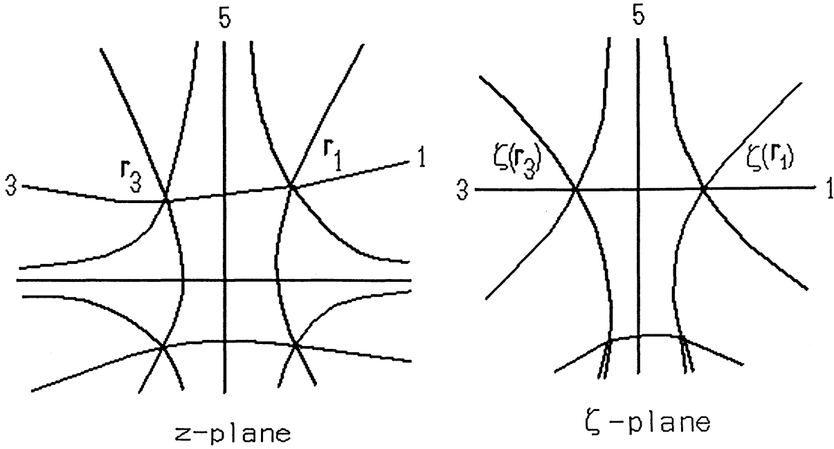
図6 ζ-平面上の様子
