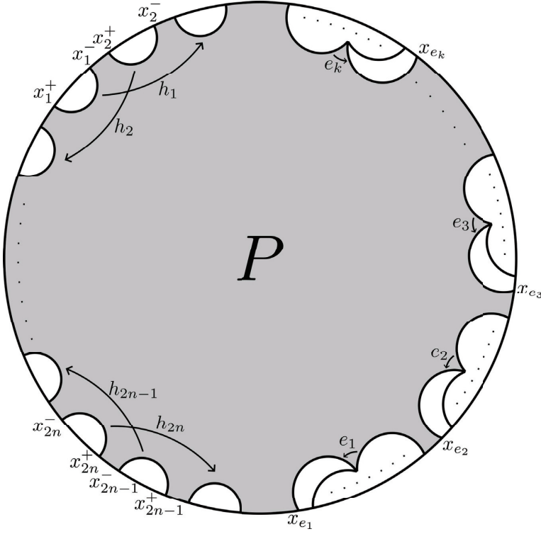
図 1 \mathbb{H}^2 上の G による作用
