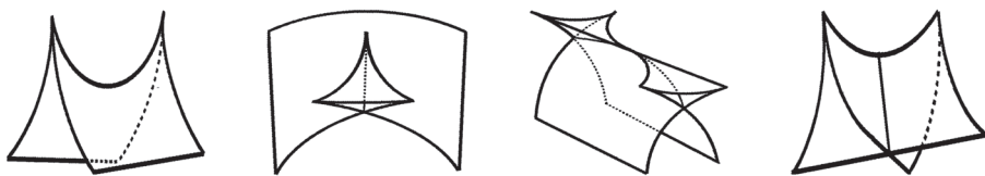
図 1: 左から, カスプ縁, 燕尾, Mond 曲面, 閉じた笠
