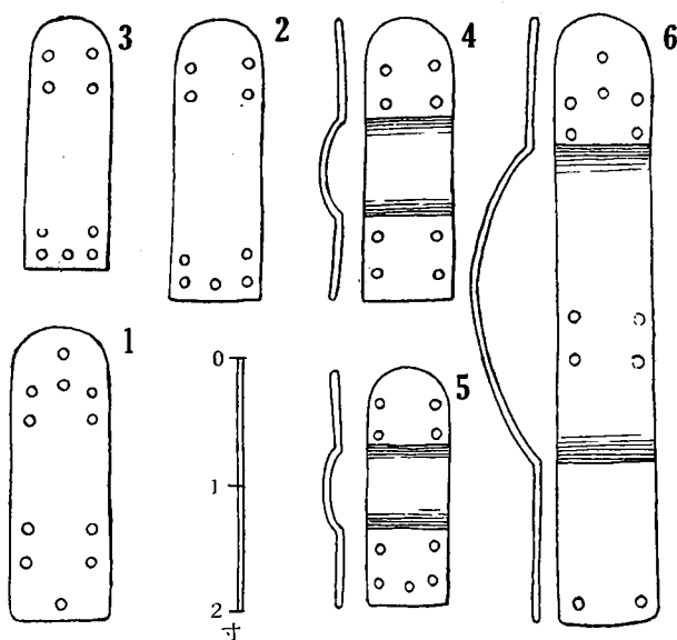
第二十三圖 挂甲小札形状圖 (Fig. 23)
