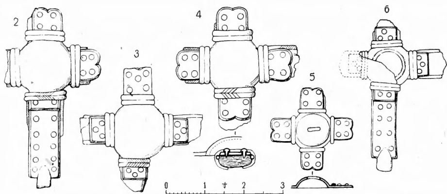
第二十五圖 十字形雲珠實測圖 (Fig. 25)
