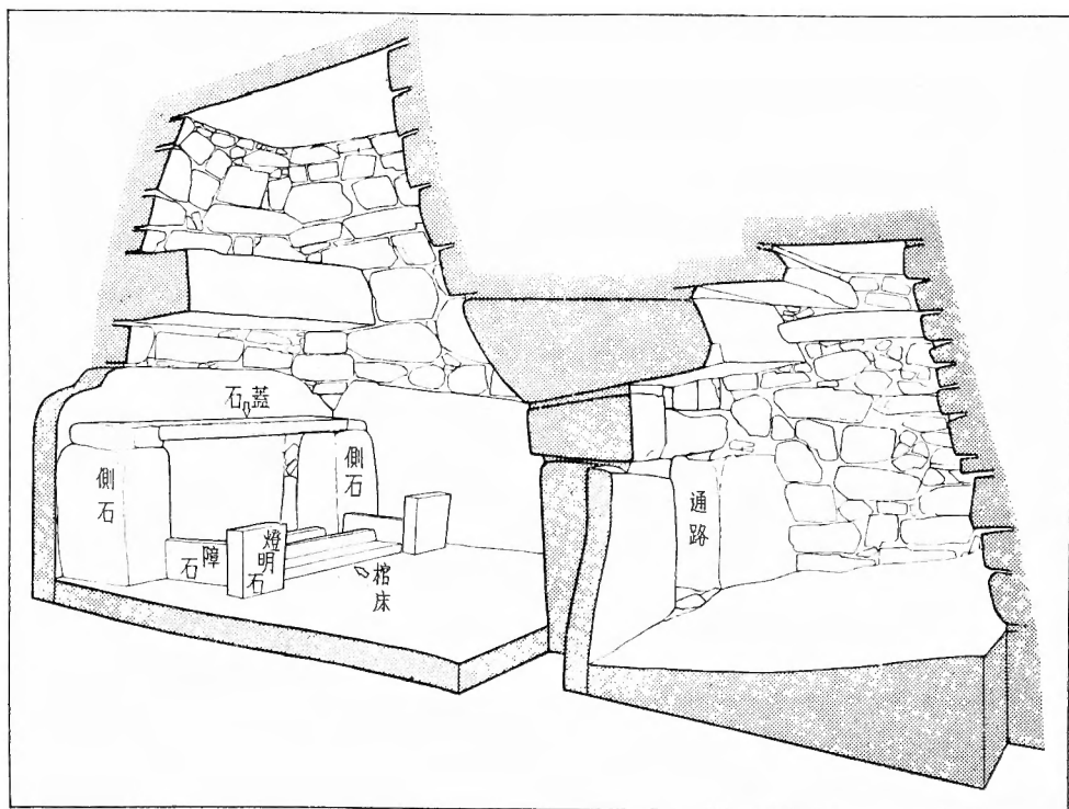
第十二圖 王塚古墳石室透視圖 (Fig. 12.)
