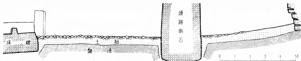
第十五圖 石室底面詳細圖 (Fig. 15.)
