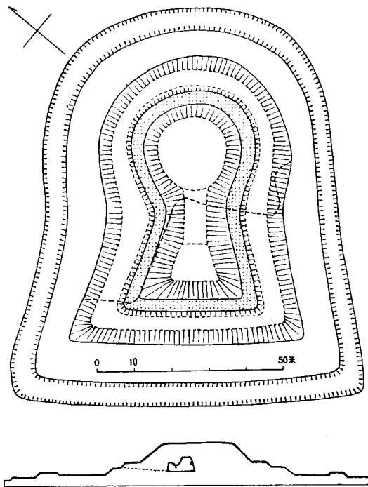
第九圖 王塚古墳外形復原試圖 (Fig. 9.)
