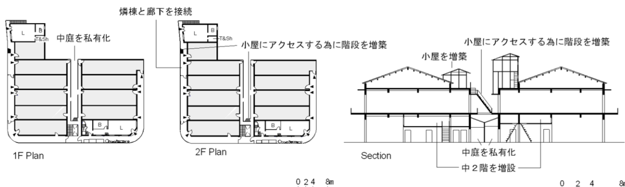
図 2-34 増改築の事例 1
