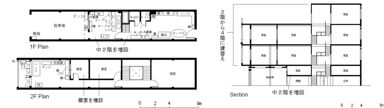
図 2-36 増改築の事例3
