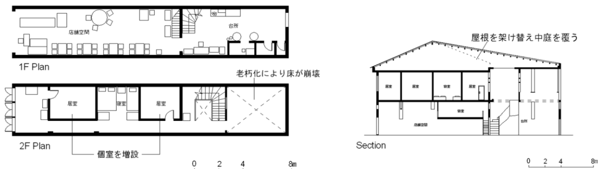
図 2-35 増改築の事例 2
