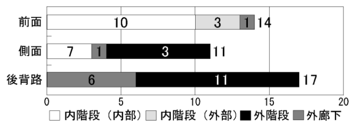
図 2-21 17 番街区の住戸経路
