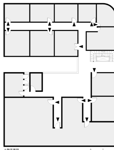
図 2-31 中廊下型
