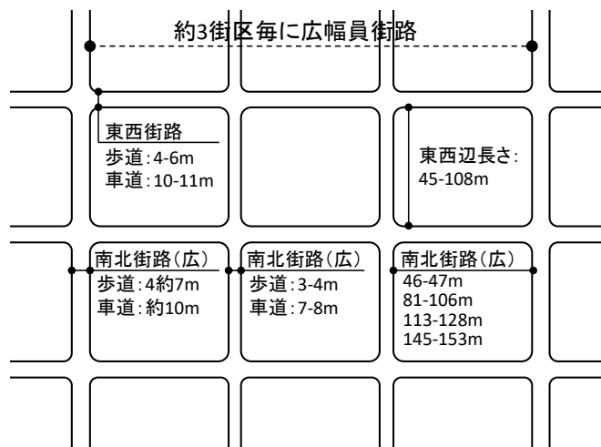
図 2-14 街路幅員と街区規模の基本型
