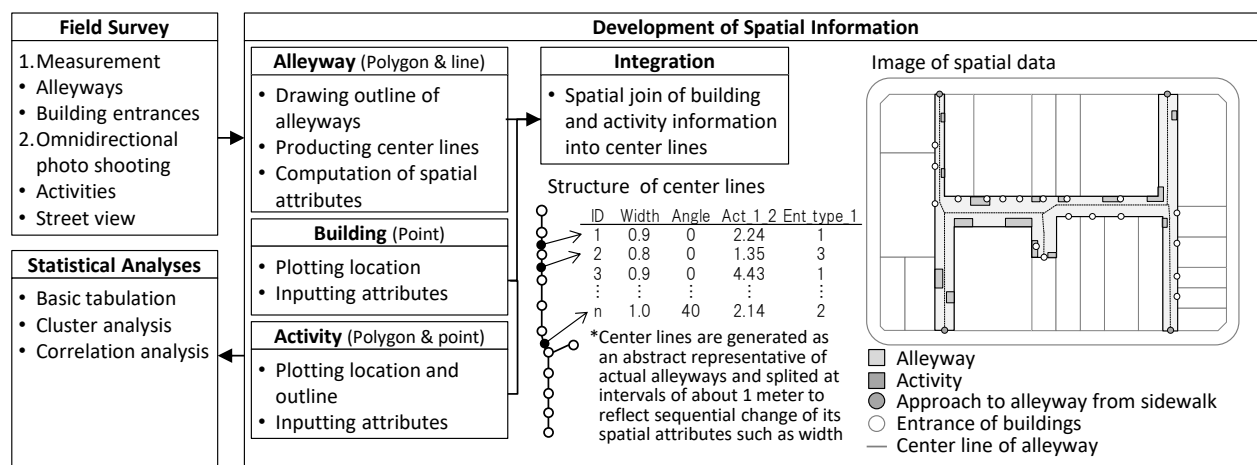
図 4-2 空間情報 DB の生成プロセス
