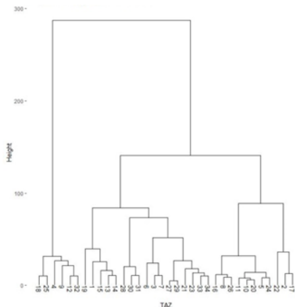
図 3-3 中心核のデンドログラム
