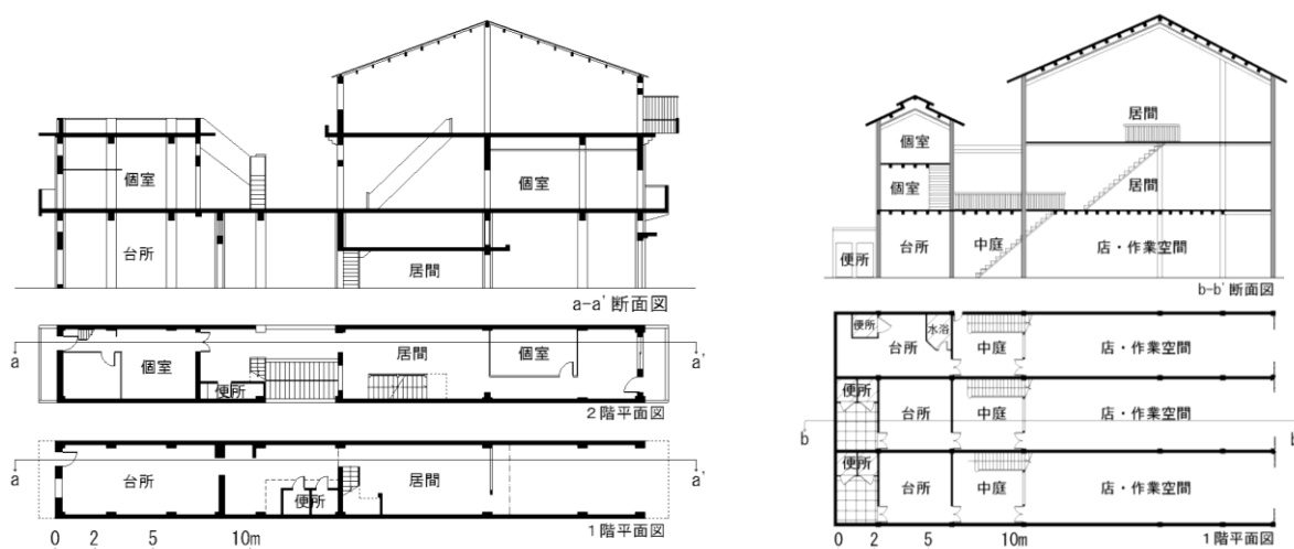
図 2-11 低層二階建てのショップハウス
