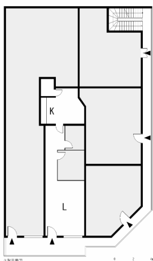
図 2-29 片廊下型
