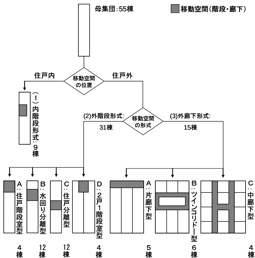
図 2-23 ショップハウスの空間類型
