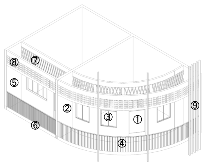
図 2-44 ファサードの構成要素
