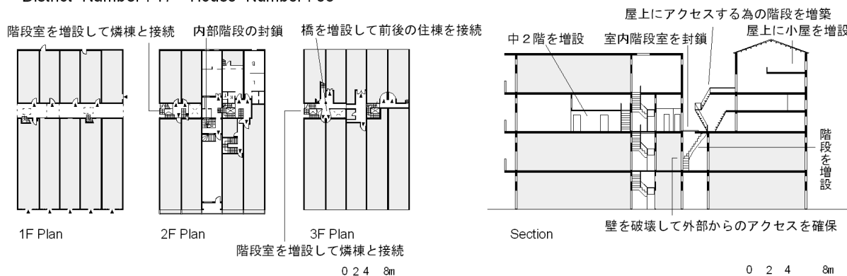
図 2-37 増改築の事例4
