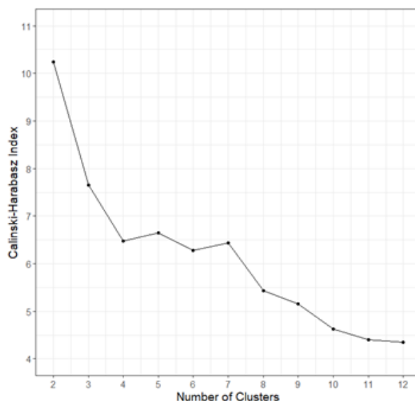
図 3-4 Calinski-Harabasz 指標の分布
