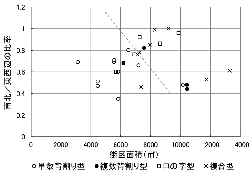
図 2-18 宅地割と街区規模
