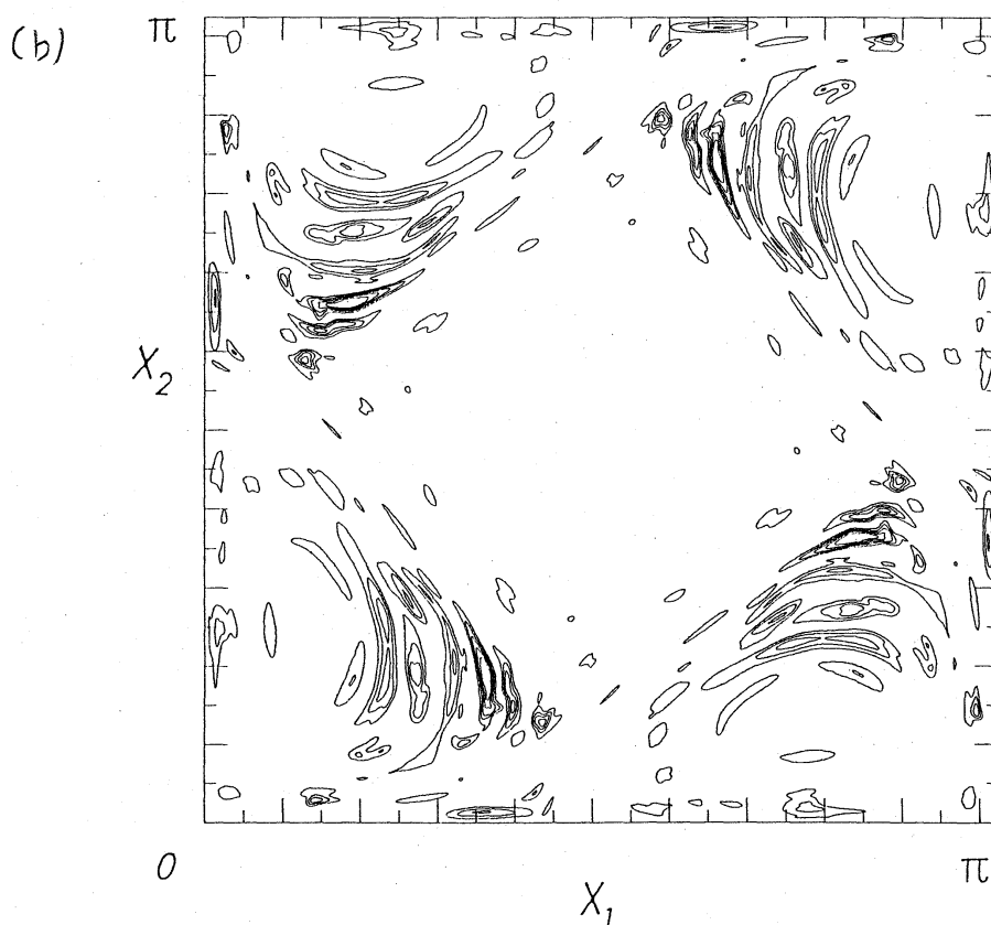
図 11 エネルギーの空間的局在 (Case I, t=12 )
