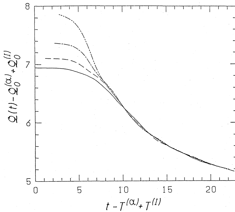
図4 エンストロフー減衰曲線
