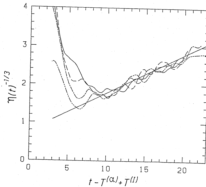
図13 \eta(t)^{-1/3} の時間変化
