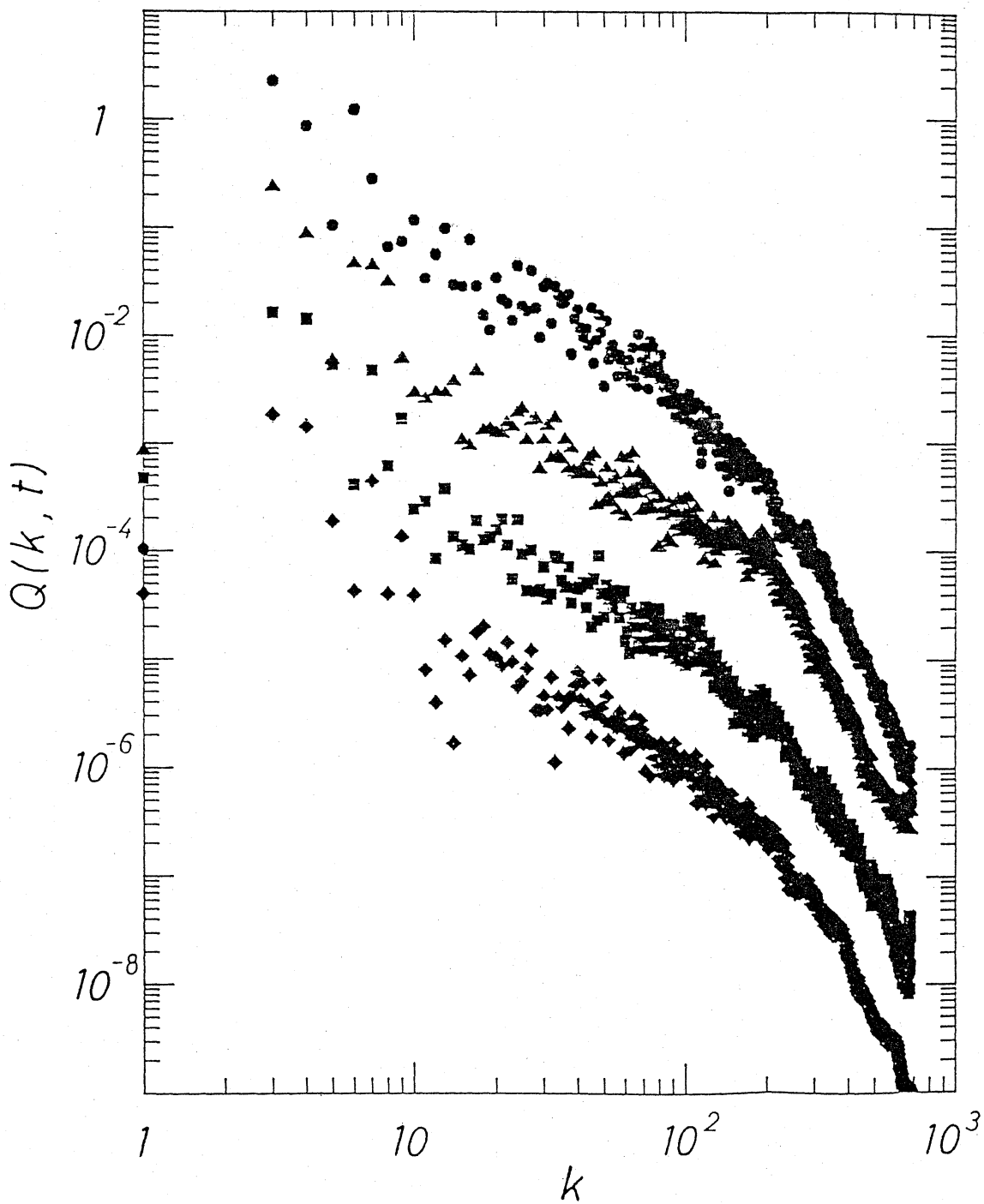
図 7 エンストロフィースペクトル (Case II)
