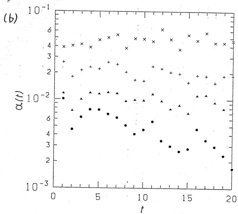
図8 n(t) 及び \alpha(t) の時間変化
