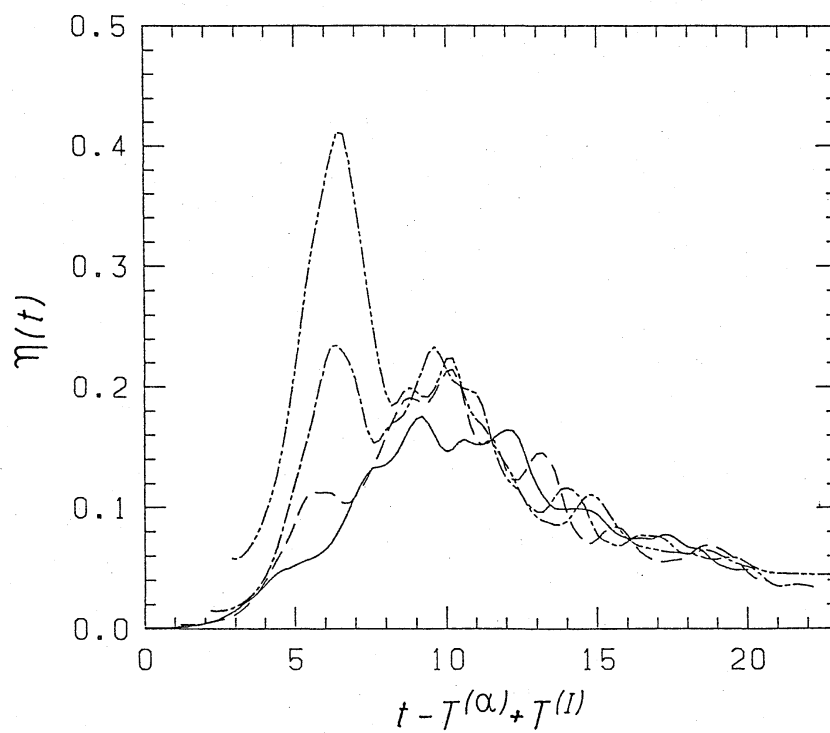
図5 エンストロフー散逸率
