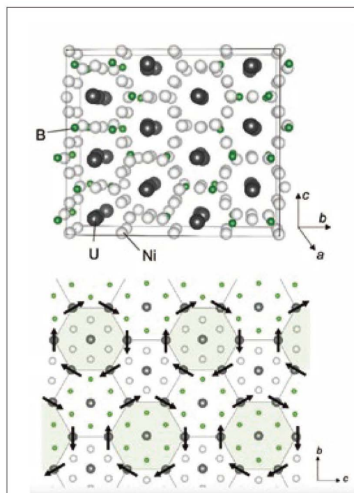
図1 ウラン化合物 (UNi 4 B) の渦状の結晶構造 (上) と磁気構造 (下)
