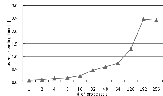
図 11 ファイル出力時間 (Weak Scaling)
