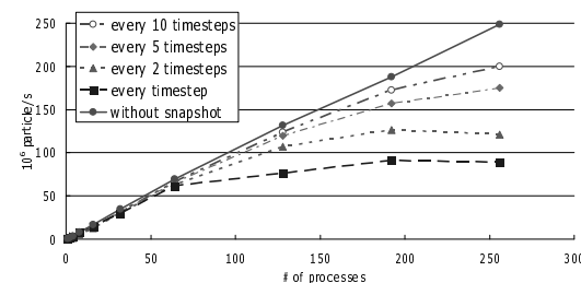
図 10 ファイル出力と性能の関係 (Strong Scaling)
