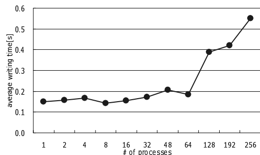
図 12 ファイル出力時間 (Strong Scaling) Fig. 12 Time to Output a Snapshot in Strong Scaling Simulation
