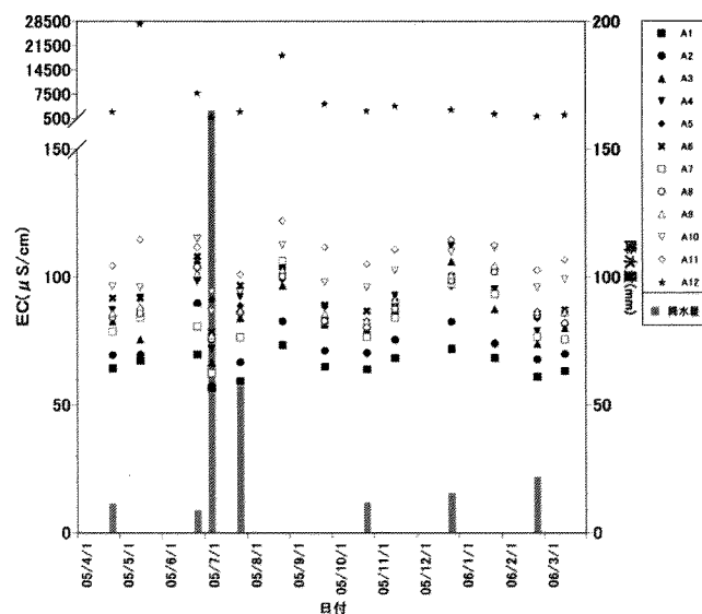
図-3 各測定日ごとの EC と先行降雨量の関係 点は採水時の各地点の EC, 棒は先行降雨を示す
