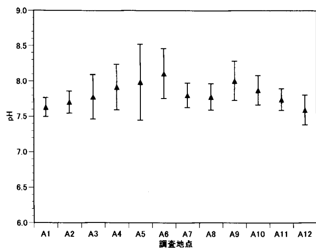
図-4 各地点の年間の平均 pH
