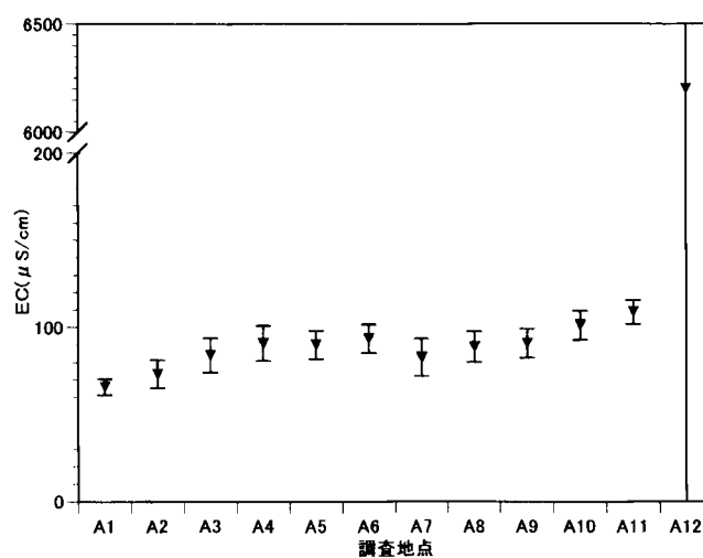
図-5 各地点の年間の平均 EC
