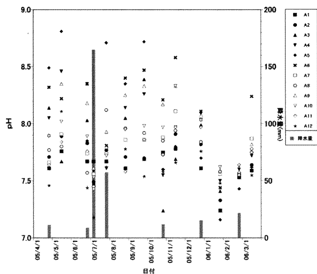
図-2 各測定日ごとの pH と先行降雨量の関係 点は採水時の各地点の pH, 棒は先行降雨を示す
