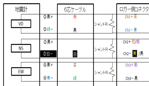
図3 配線図
