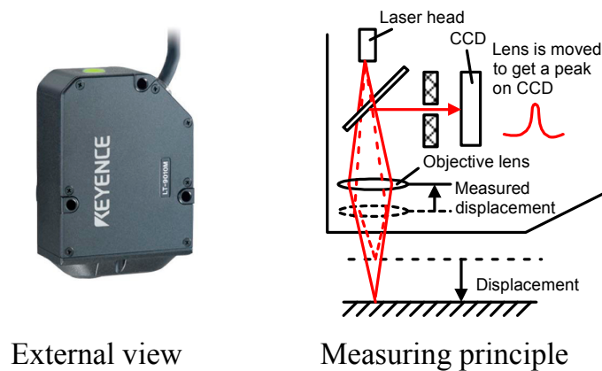
(d) Confocal type (LT-9010MS)
