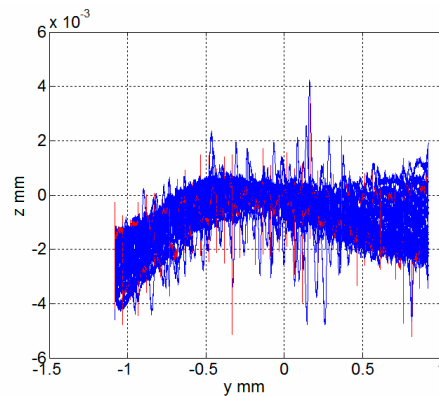
(d) Profile measurement error along Y-direction
