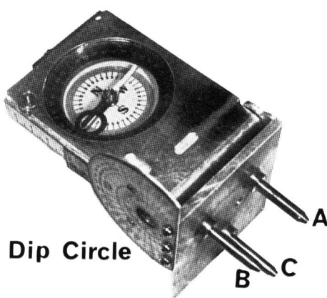
Fig. 6. Orientation apparatus.
