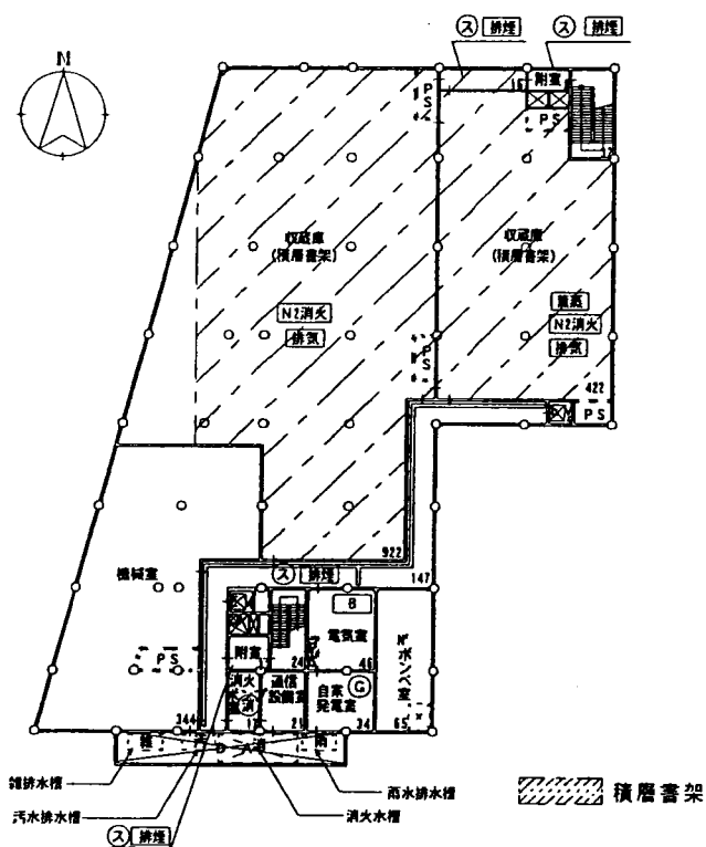
地下3 階平面図
