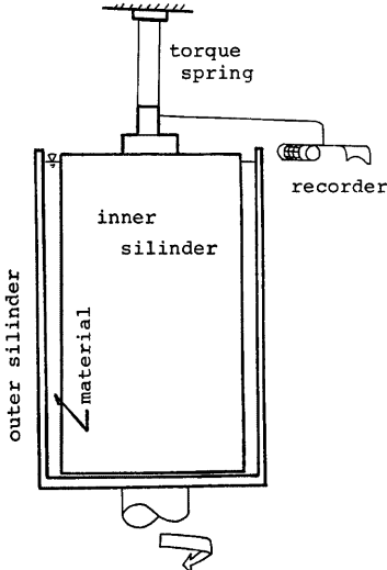
Fig. 11 Viscometer
