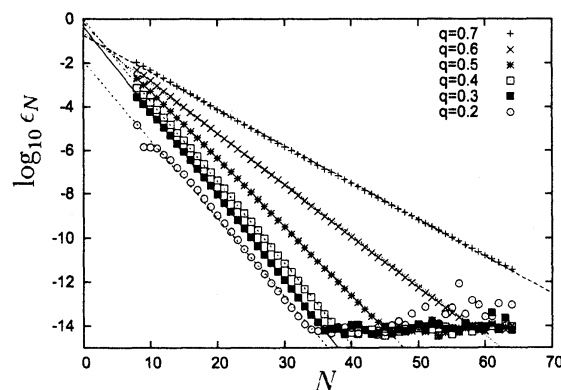
図 2: 2次元円外領域におけるポテンシャル問題に対する代用電荷法の誤差.
