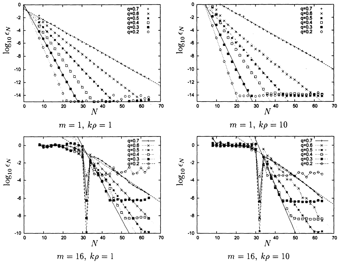
図 4: 境界データ f^{(1)} の波動問題に対する代用電荷法の誤差。
