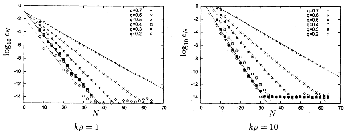
図 5: 境界データ f^{(II)} の波動問題に対する代用電荷法の誤差.
