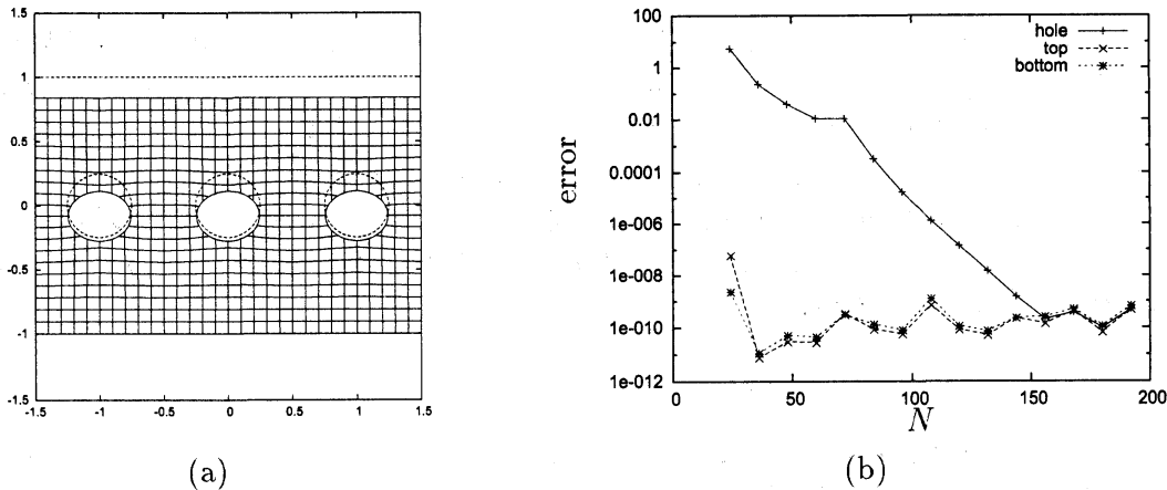
図 3: (a)1 次元周期的に並ぶ円孔を持つ 2 次元弾性体. 上面に一様に圧力を加え, 下面を固定している. そして, 円孔境界には応力は働いていない. (b)1 次元周期的円孔列をもつ 2 次元弾性体の問題に対する代用電荷法の誤差. (a), (b) ともに [8] より引用.
