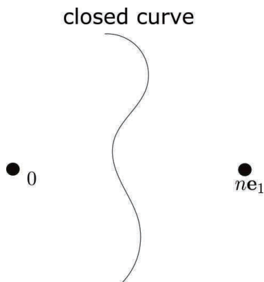
FIGURE 3. 二次元で大偏差が起こる例
