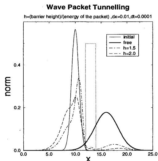
図 24: 波束の運動 2
