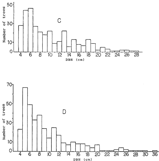
図 4.2 プロット別の直径階別本数分布
