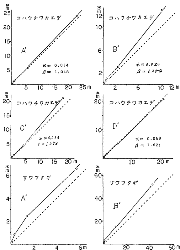
図 8.2 樹種別プロット別の分布様式( m^* - m 関係)
