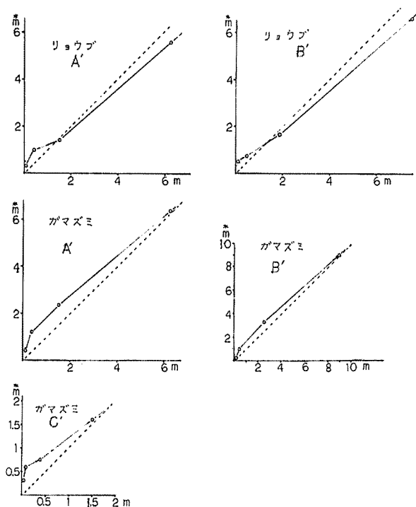
図 8.1 樹種別プロット別の分布様式 ( \bar{m}-m 関係)
