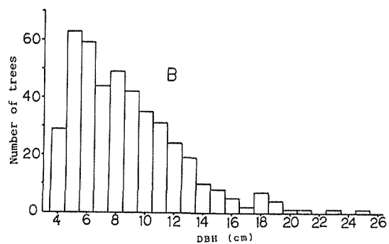
図 4.1 プロット別の直径階別本数分布
