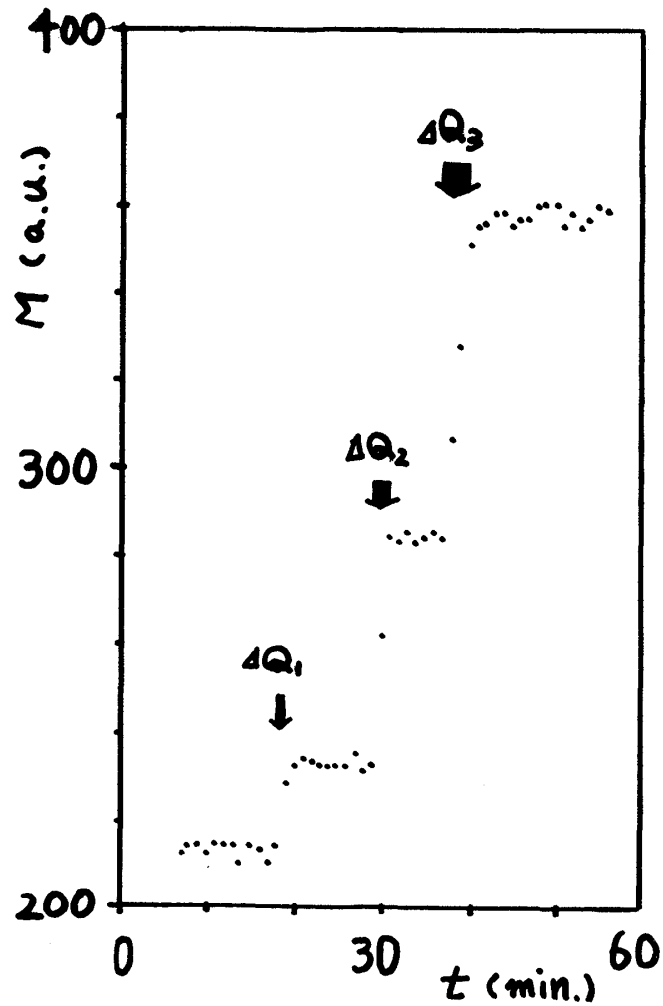
図2. 熱注入による磁化の変化 T = 7.50 \text{ mK}
