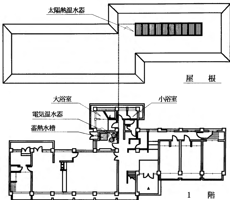
図1 浴室および浴室給湯設備の配置
