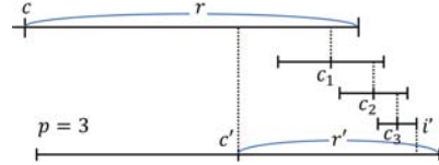
図 7 補題 6 における, 極大回文と関数 skip の返回值 i_2, p との関係の例 図の関係においては, i_2 = i' および p = 3 を返し, このとき, Stack は空である.
