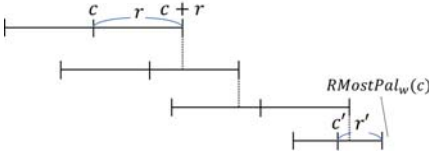
図 2: RMostPal_w(c) と極大回文との関係
