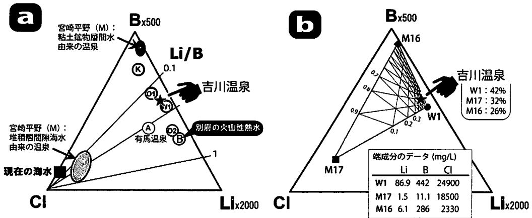
図 3 (a) スラブ脱水流体由来する温泉 (K, W1, O1, O2, A) とそれに類似する吉川温泉の Li-B-Cl 組成, (b) 起源流体 (堆積層間隙海水, 粘土鉱物層間水, 変成脱水流体) のモデル温泉 (M17, M16 と W1) を端成分として混合して生成する流体の Li-B-Cl 組成範囲
