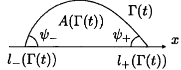
図 1: 解の形状
