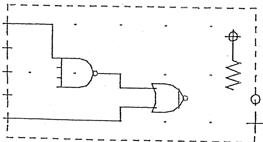
図5. 回路図の例
