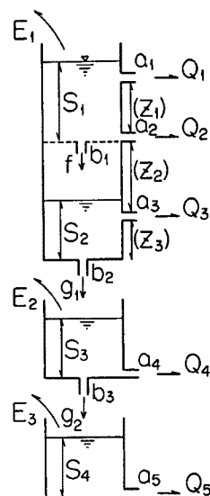
Fig. 1. LST Model.
