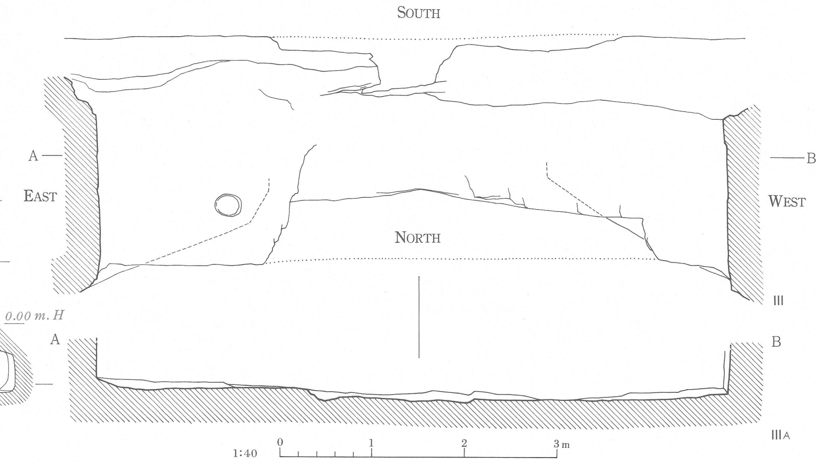
III PLAN OF WINDOW FLOOR, IIIA SECTION 明り窓床平面 断面図
