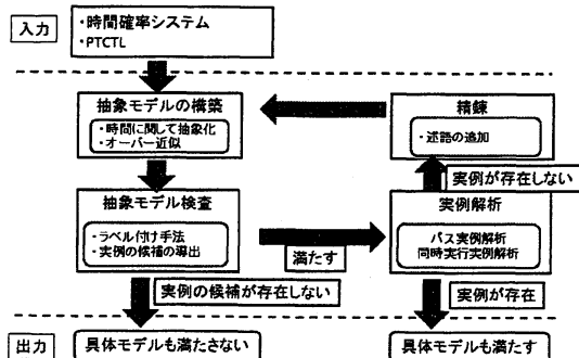
図4: 確率時間 WiGAR による検証の流れ
