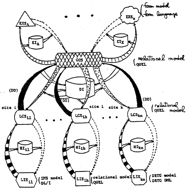
図2.2 四層スカープ構造
