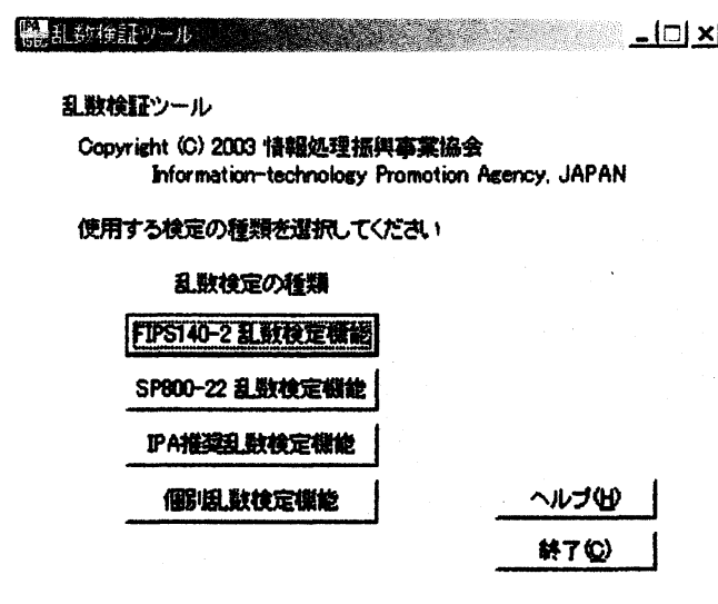
図 1: 初期画面
