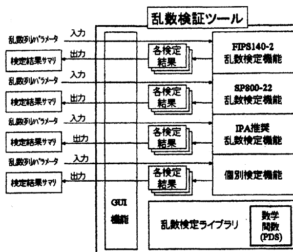
図 3: 乱数検定ツールの機能関連図
