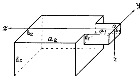
第1圖 棚であり灣である小湖海の模型
