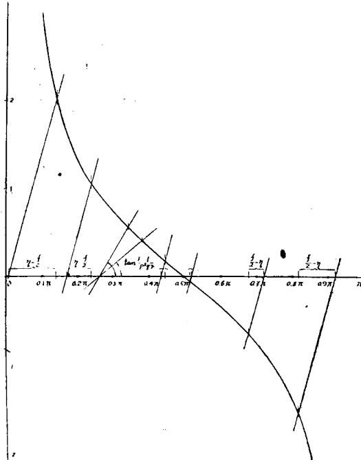
第2圖 週期方程式の根
