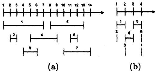
図 2: 冗長な区間表現と対応するコンパクトな区間表現
