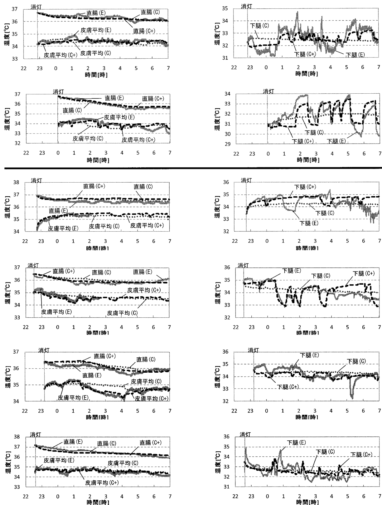
図7 各部温度(上から夏期第1回, 第2回, 冬期第1回, 第2回, 第3回, 第4回)
