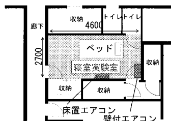
図1 実験室見取り図
