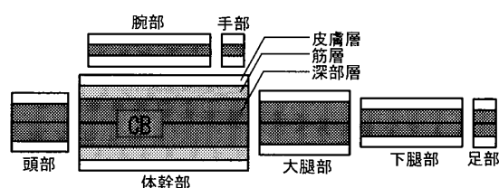
図6 人体熱モデルの模式図
