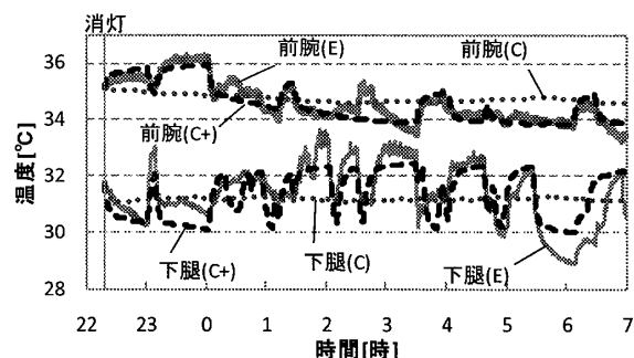
図5 各部位の温度
