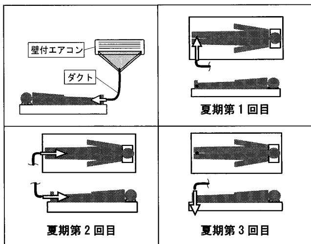
図3 局所冷暖房の模式図(左上)と 夏期実験における送風ダクトの位置と向き
