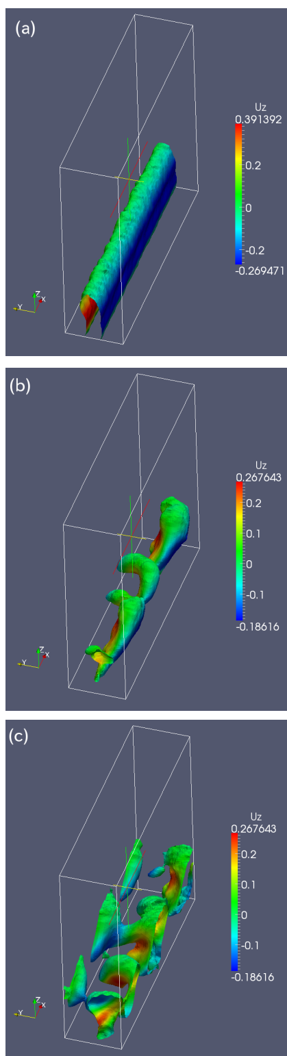
図 5.10: 上から時刻 t=300 (s), 750 (s), 850 (s) における圧力 -0.03 (Pa) の等値面. 管の内部は低圧渦になっている. 面についている色は鉛直流速を表す.
