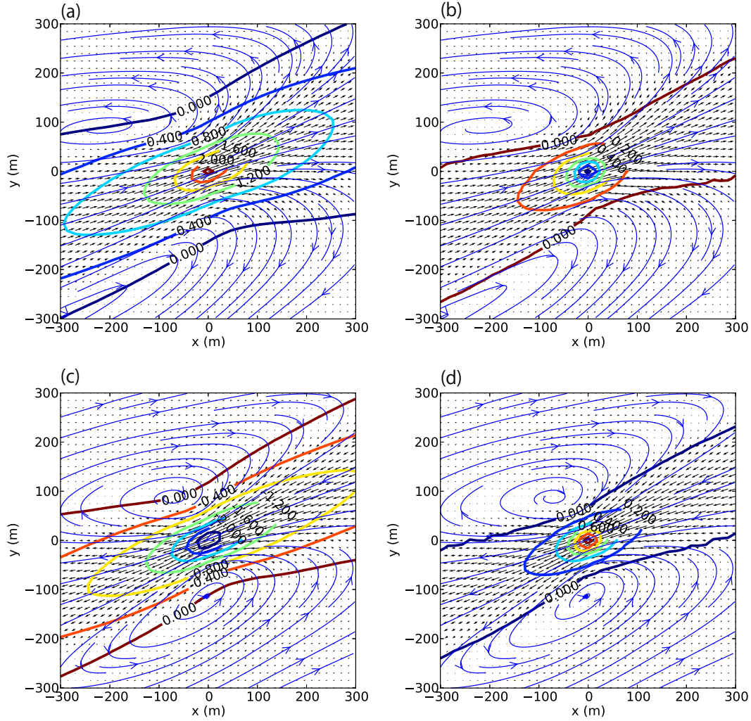
図 2.12: コンディショナルサンプリングで得られた水平速度 (a),(c) と鉛直速度 (b),(d) の水平断面分布. (a),(b) がスweep (水平流が高速で下降流), (c),(d) がイジェクション (水平流が低速で上昇流) を条件に課したときの分布. 矢印と流線は水平風速の分布を示している. 等値線についたラベルは速度の値である.
