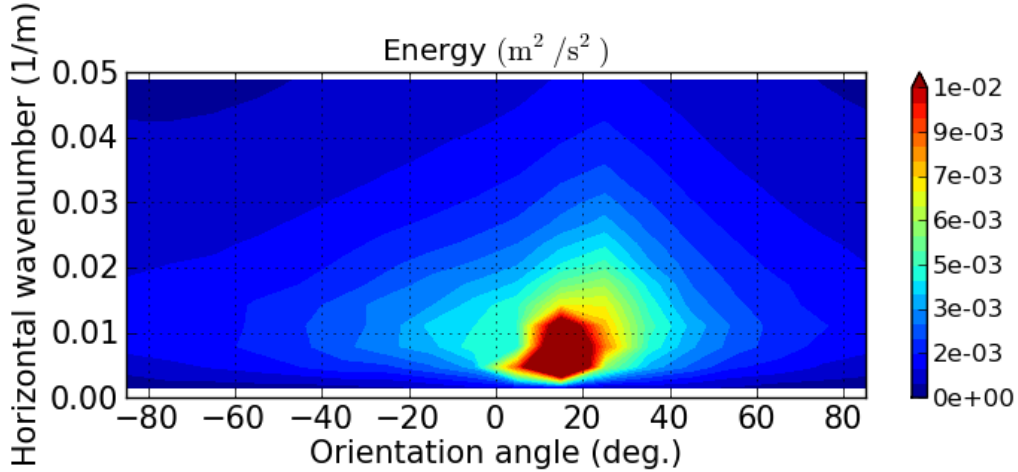
図 2.15: フィルタリングによって抽出された摂動が持つ運動エネルギー (高度が 0 から 500m までの平均値) の水平波数 (縦軸) と地衡風とのなす角 (横軸) へのパラメータ依存性。値が低い領域の高低を見やすくするために大きな値の等値線を省いてある。運動エネルギーが最大の摂動のパラメータは \alpha = 0.0047 (1/m), \epsilon = 15^\circ で最大値は 1.9 \times 10^{-2} (\text{m}^2/\text{s}^2) である。
