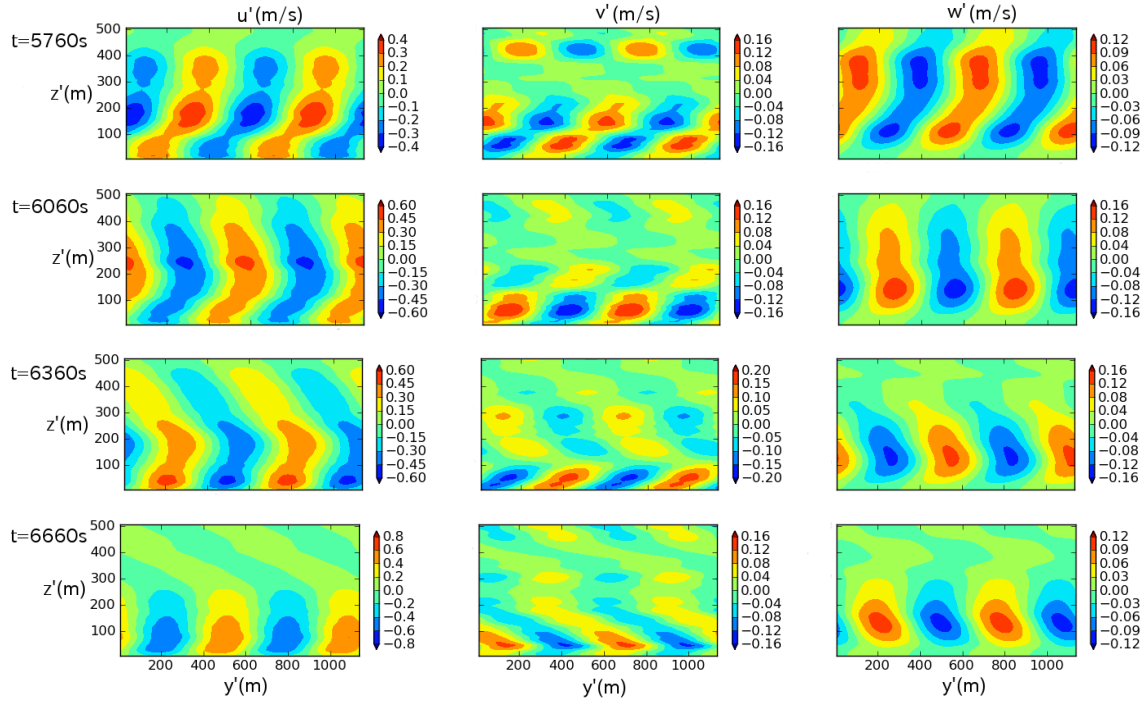
図 2.21: ケース 18 の数値実験で得られたストリーク構造の速度の 3 成分 ( u', v', w' ) の y' - z' 断面での時間変化, 時刻は上から t=5760\text{s} , 6060\text{s} , 6360\text{s} , 6660\text{s} である。フィルタリングを行っているためすべての x' で摂動のパターンは同一である。
