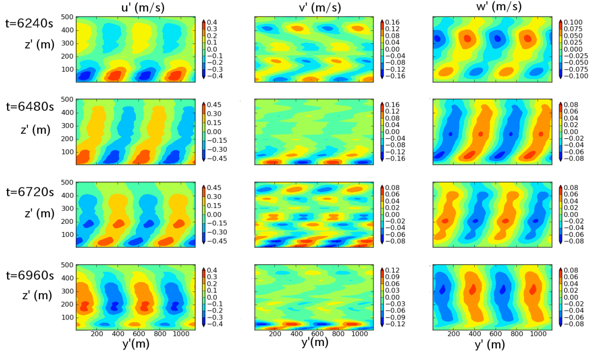
図 A.2: ケース 6: 時刻 t=6240s , 6480s , 6720s , 6960s . 図の設定は図 2.21 と同じである.
