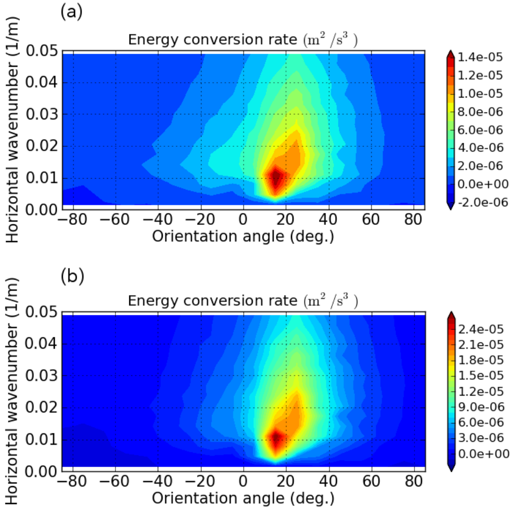
図 2.16: フィルタリングによって抽出された摂動に平均流から変換される運動エネルギーの量の水平波数 (縦軸) と地衡風とのなす角 (横軸) へのパラメータ依存性. 平均領域は地面から高度 500m まで (a) と 高度 250m まで (b). エネルギー変換量の最大の摂動のパラメータは (a) は \alpha = 0.011 \text{ (1/m)} , \epsilon = 15^\circ で最大値が 1.5 \times 10^{-5} , (b) は \alpha = 0.011 \text{ (1/m)} , \epsilon = 15^\circ で最大値が 2.7 \times 10^{-5} (\text{m}^2/\text{s}^3) である.
