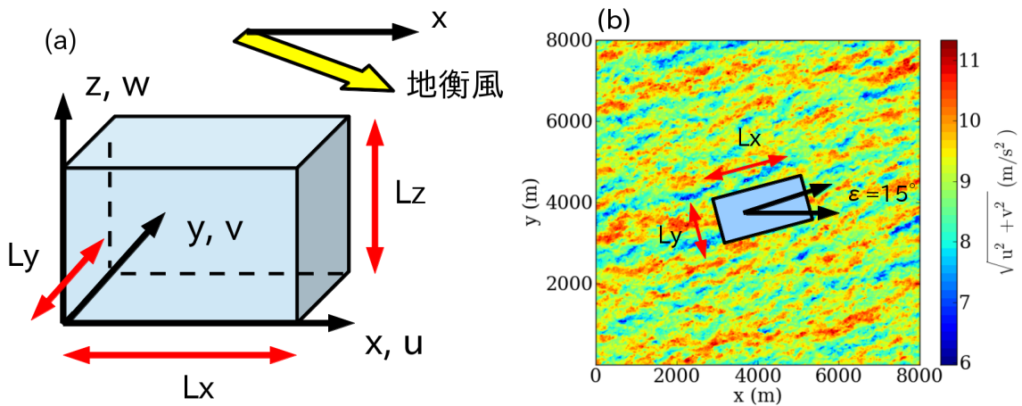
図 2.18: (a) ミニマル領域 LES の計算領域. 地衡風の方角を x 軸の方角から時計回りに 15^\circ 度回転させている. (b) ミニマル領域 LES の初期条件の決定方法. 大規模領域 LES の水平領域 (大きさが x 軸方向に 8000\text{m} , y 軸方向に 8000\text{m} ) から, x 軸方向に L_x で y 軸方向に L_y のミニマル計算領域を切り出す. 2つの領域の中心位置は同じにした.
