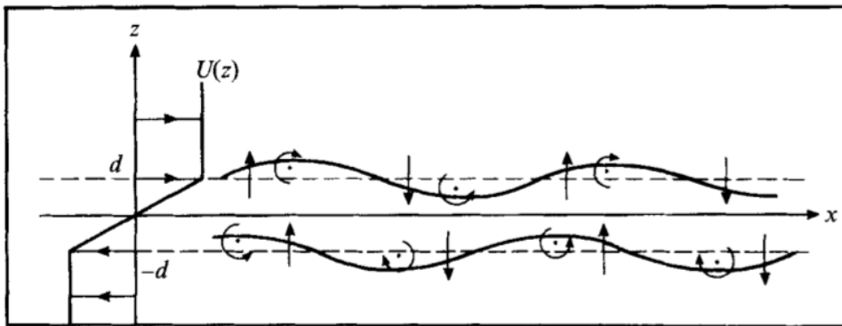
図 3.1: 波の共鳴によって引き起こされる変曲点不安定の概念図。変曲点を持つ風速プロファイルを区分的線形なプロファイルに置き換えて、エッジ ( z = d, -d の地点) の所に捕捉されたロスビー波の共鳴により不安定が起こることを説明した。?より引用。
