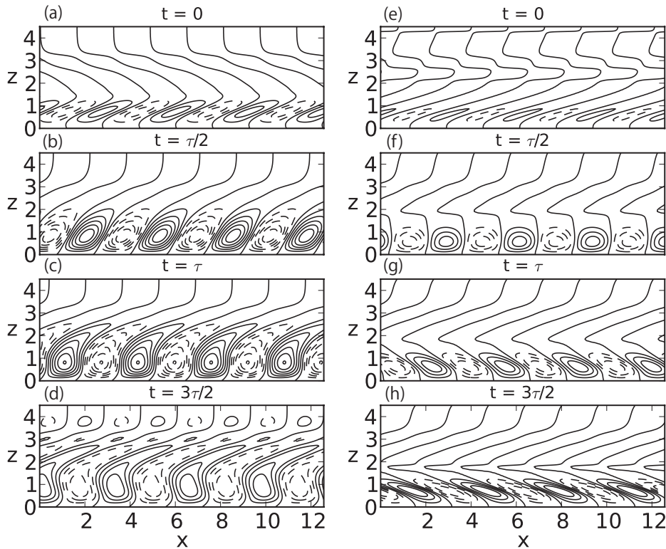
図 3.15: 最適化時間 \tau = 15 で最大のエネルギーノルム増幅率を示す最適摂動 ( \alpha = 1.94, \epsilon = 33.1^\circ ) の流線関数 (a)–(d) と軸方向速度 (e)–(h) の時間変化. 上から時刻 t = 0, 0.5\tau, \tau, 1.5\tau における分布を示す. 等値線の間隔は流線関数はすべて 0.1, 軸方向速度は上から 0.1, 1, 2, 2 となっている.
