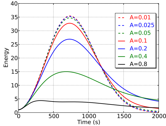
図 5.3: 様々な振幅での非線形時間発展をした時の最適摂動のエネルギーの時間変化. t=0 での全エネルギーを 1 として規格化してある.
