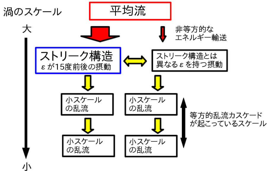
図 2.25: エクマン層における乱流のエネルギーカスケードの概念図. 平均流が持つ運動エネルギーが小スケールの渦の運動エネルギーに変換されていく様子を示している. 平均流からスケールの大きな渦にエネルギーが移される (赤矢印) 際には, ストリーク構造に対応する特定の向き ( \epsilon \sim 15^\circ ) を持つ擾乱に大部分のエネルギーが供給されており, エネルギーカスケードが非等方性を示す. より小スケールの乱流では等方的なエネルギーカスケード (黄矢印) が実現している.
