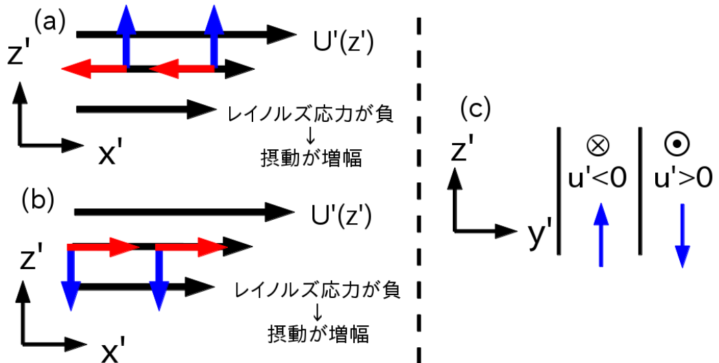
図 2.23: ロールメカニズムの概念図. (a) と (b) が x' - z' 断面, (c) が y' - z' 断面を示している. (a) と (b) での黒矢印は平均流 U'(z') を表し, 青線が擾乱の鉛直成分 w' , 赤線が擾乱の水平成分 u' を示している. (a) では上昇流とそれに伴う水平低速流によってレイノルズ応力 u'w' が負になり摂動が発達する様子を, (b) では下降流と水平高速流の場合で同様にレイノルズ応力が負となり摂動は発達する様子を示している. 擾乱は x 軸方向には一様であり, (c) に示されているように y' 軸方向に位相が変化している.
