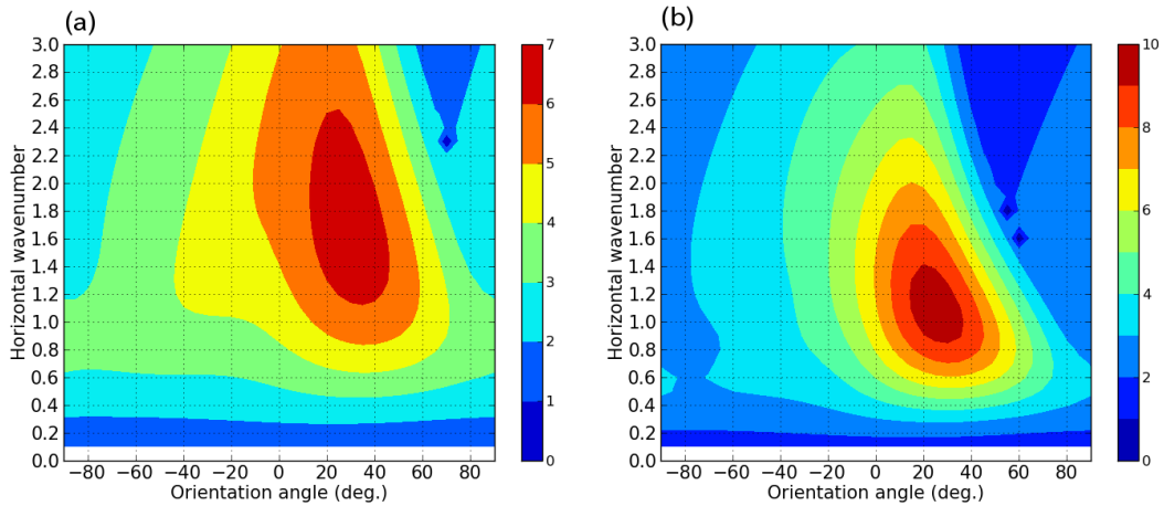
図 3.9: 最適摂動のエネルギーノルム増幅率のパラメータ (水平波数 \alpha と地衡風とのなす角 \epsilon ) 依存性. (a):最適化時間 \tau = 15 , (b):最適化時間 \tau = 25 , それぞれ最大値を取るのは (a) は \alpha = 1.68, \epsilon = 29.7^\circ の時で増大率は 6.6011, (b) は \alpha = 1.085, \epsilon = 25.3^\circ の時で増幅率は 9.5960 である.
