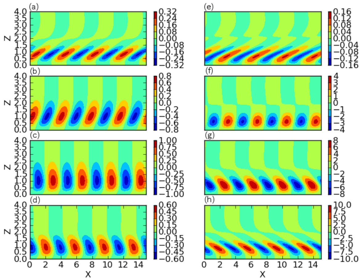
図 3.10: 最適化時間 \tau = 15 で最大のエネルギーノルム増幅率を示す最適摂動の流線関数 (a)-(d) と軸方向速度 (e)-(f) の時間変化．水平波長 \alpha=1.68 ，地衡風とのなす角 \epsilon = 29.7^\circ ．上から時刻 t = 0, 0.5\tau, \tau, 1.5\tau における分布を示す．値のスケールが図ごとに異なる点に注意が必要である．
