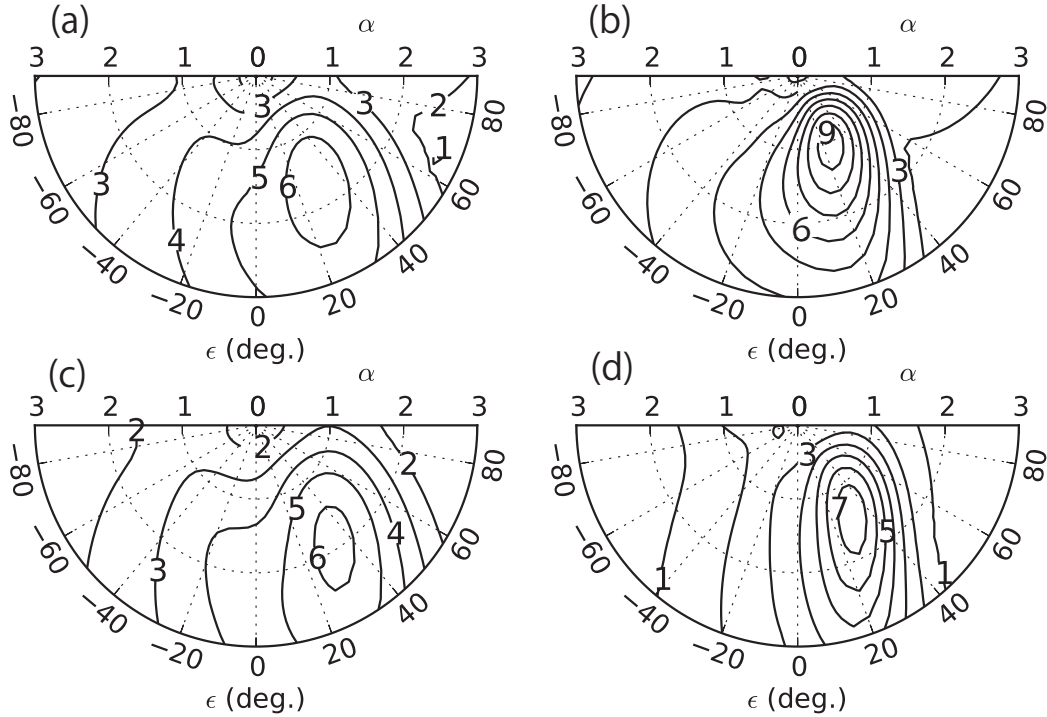
図 3.14: 最適摂動のエネルギーノルムの増幅率の水平波数 \alpha と地衡風とのなす角 \epsilon に関するパラメータ依存性. (a), (c):最適化時間 \tau = 15 , (b), (d):最適化時間 \tau = 25 , (a), (b) は図 3.9 と同じ結果で逆転層が無い場合の最適摂動の結果. (c), (d) は逆転層高度が z_i = 3.0 の時の最適摂動の結果. それぞれ最大値を取るのは (a) は \alpha = 1.68, \epsilon = 29.7^\circ の時で増幅率は 6.6011, (b) は \alpha = 1.085, \epsilon = 25.3^\circ の時で増幅率は 9.5960, (c) は \alpha = 1.94, \epsilon = 33.1^\circ の時で増幅率は 6.3216, (d) は \alpha = 1.48, \epsilon = 30.5^\circ の時で増幅率は 7.6221.
