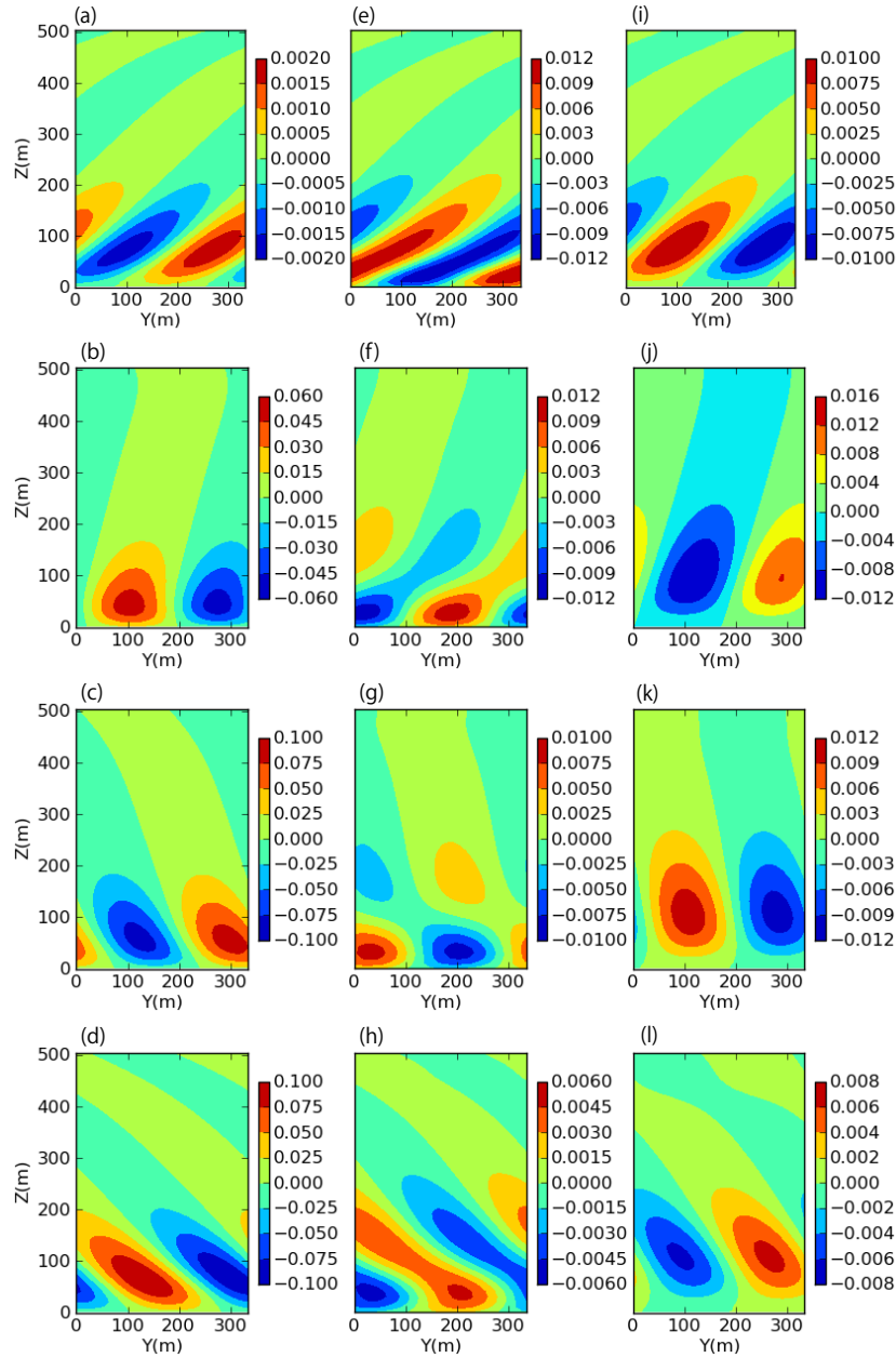
図 5.5: 振幅 A = 0.01 の最適摂動 (最適化時間 500s) の摂動成分の時間変化. (a) から (d) が u , (e) から (h) が v , (i) から (l) が w の分布を表している. 上から (a),(e),(i) が t=0s , (b),(f),(j) が t=250s , (c),(g),(k) が t=500s , (d),(h),(l) が t=750s である.
