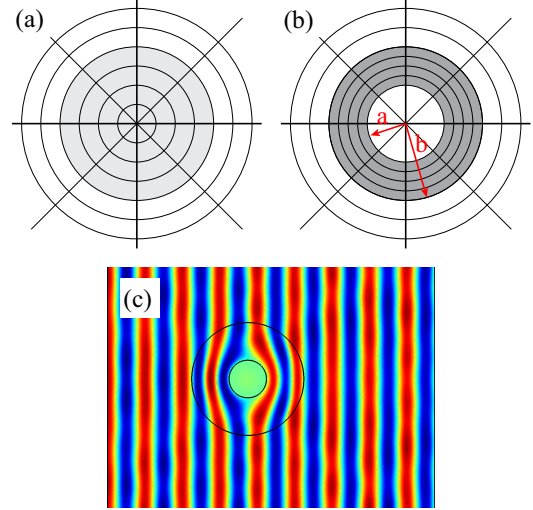
図 9: 透明マントの原理. (a) 元の系. (b) 写像後の系. (c) シミュレーション結果.
