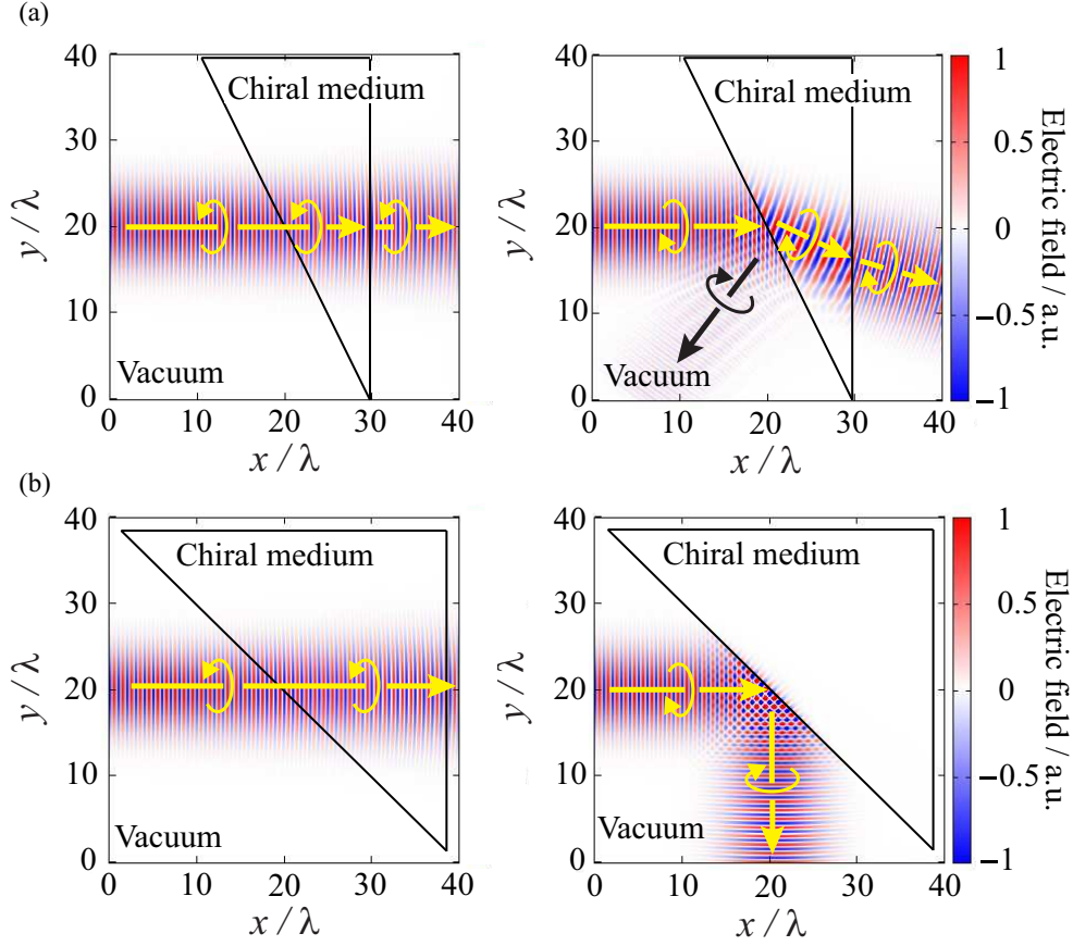
図 7: 円偏光無反射現象を利用した円偏光ビームスプリッター. (a) 入射角 < 臨界角, (b) 入射角 > 臨界角のときの左円偏光, 右円偏光の伝搬.
