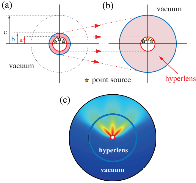
図 10: ハイパーレンズを実現する写像. (a) 元の系. (b) 写像後の系. (c) シミュレーション結果.
