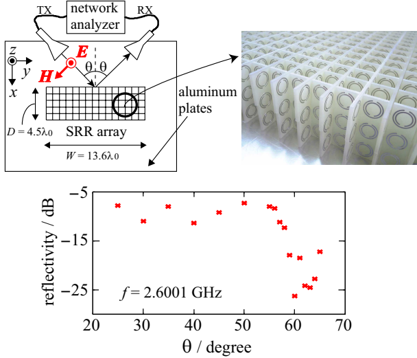
図 3: マイクロ波領域における s 波ブルースタ現象の実験.
