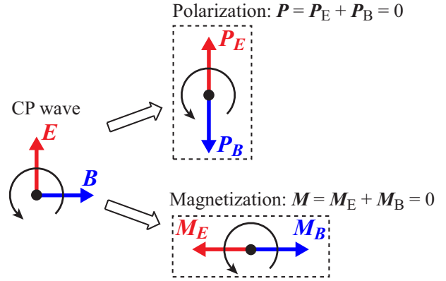
図 6: 円偏光に対する無反射条件の物理的意味。
