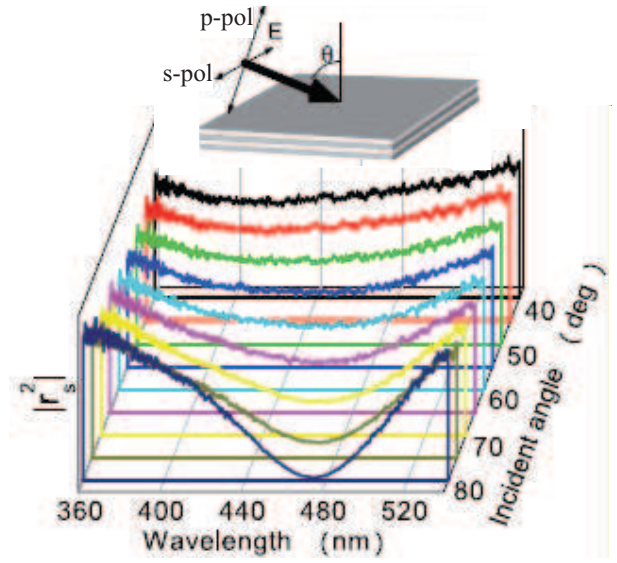
図 4: 光領域における s 波ブルースタ現象の観測結果.
