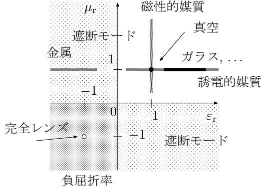
図 1: 誘電率-透磁率平面
