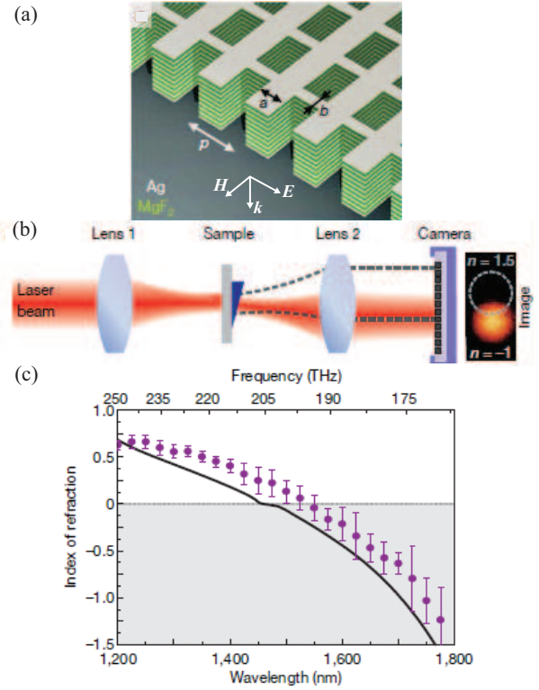
図 2: (a) 負屈折率 ( \lambda \sim 1.5 \mu\text{m} ) のための網目構造. a = 565 \text{ nm} , b = 265 \text{ nm} , p = 860 \text{ nm} , (b) 実験系, (c) 屈折率の測定値と厳密結合波理論による計算値 (実線).
