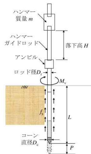
図-1 動的コーン貫入試験の概要
