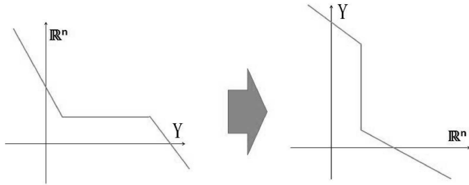
図 2: 単純な連続関数とその逆写像のグラフ
