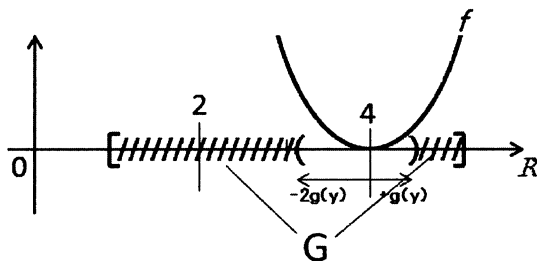
図 1: 例 3.3 の様子
