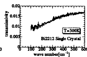
Fig.2 Bi2212 単結晶における透過率の波数依存性 ( T=300K )
