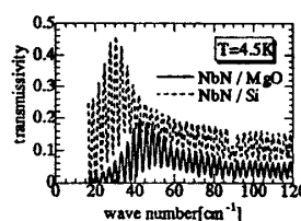
Fig.1 NbN 薄膜における透過率の波数依存性 ( T=4.5K )
