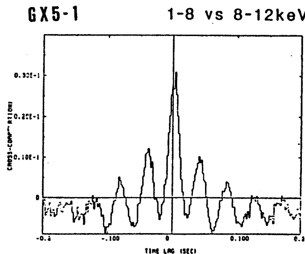
図9 GX5-1からのQPO ( \sim 20\text{Hz} ) の、二つのX線エネルギーバンド間の、cross correlation function。『ぎんが』衛星による。
