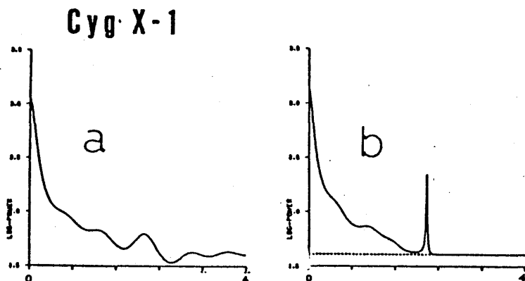
図15 ARモデルによるCyg X-1のパワースペクトル。a: 通常のARモデル、b: ポアッソノイズを考慮したARモデル。北川 1987より。
