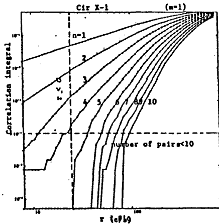
図4 Cir X-1のフレアーのライトカーブの10次元までのcorrelation integral。サンプリング間隔 m=1 の場合。典型的な量子ノイズ \sigma が半径 r より大きくなる領域（左側）と、半径内のペアの数が10以下の領域（下側）も示されている。
