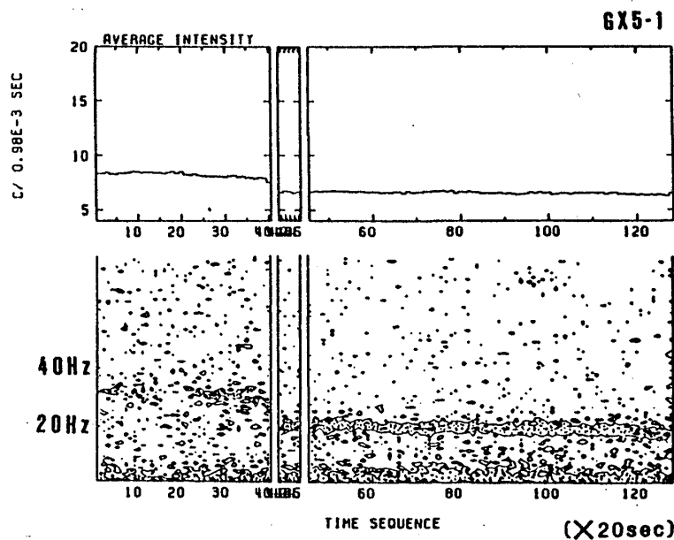
図8 LMB, GX5-1からのQPO(中心周波数=20-30Hz)。
