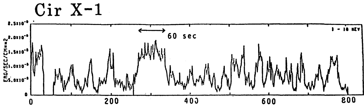
図3 『てんま』衛星が観測したCir X-1のフレアーのライトカーブ。
