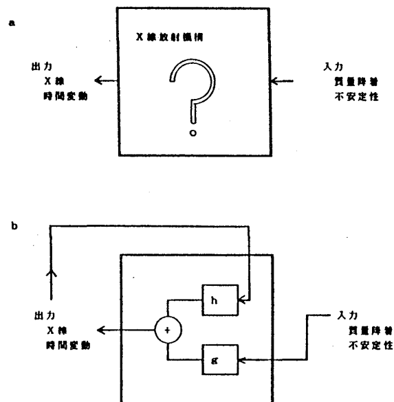
図14 a: 外乱を受けたX線時間変動のシステム。b: システムを決定論的な部分と、確立的な部分の二つの和に表わす。
