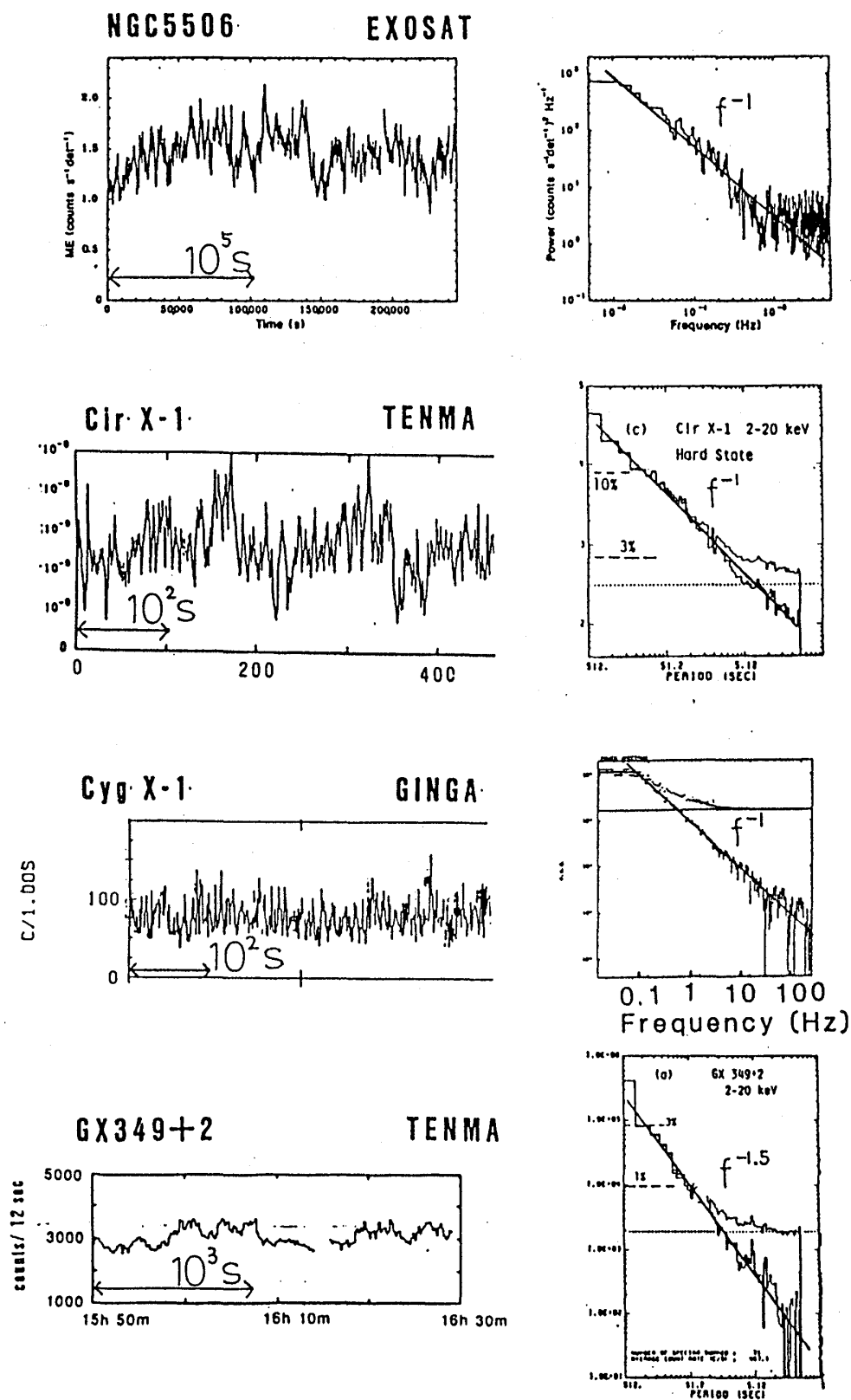
図1 セイファートII型銀河NGC5506, 中性子星を含むX線連星Cir X-1、ブラックホール候補のX線連星Cyg X-1、小質量連星X線源GX349+2のライトカーブとパワースペクトルの例。この例ではパワースペクトルがいずれも、広い周波数範囲でべき関数で表わされる。『ぎんが』衛星以外のデータは、McHardy & Czerny 1987, Makishima 1986, Ikegami 1987, Mitsuda 1984より。
