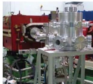
FFAG加速による材料照射試験装置
