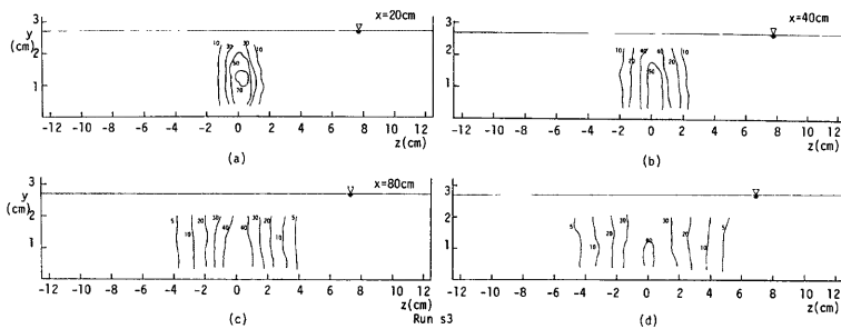
Fig. 3 (a), (b), (c), (d) Concentration distribution.
