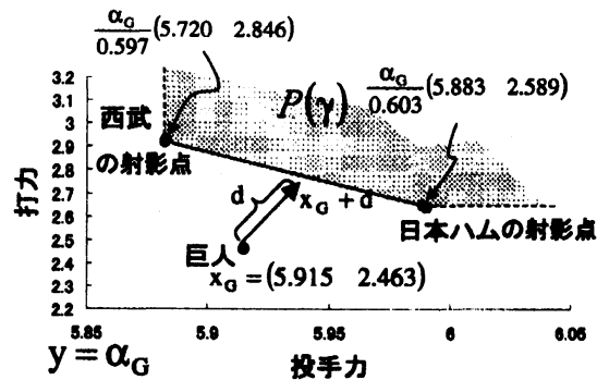
図 2: 平面 y = \alpha_G 上の P(\gamma) と巨人の戦力
