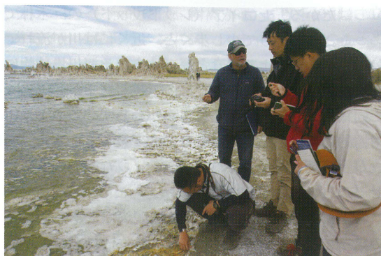
写真3. モノ湖の湖岸で炭酸カルシウムの沈殿を眺める様子。写真奥には炭酸カルシウムの柱状岩 (トゥファ) が見える。
