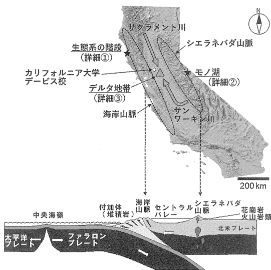
図 1. カリフォルニア州の地理（上）と過去のプレート運動の様子（下）。
