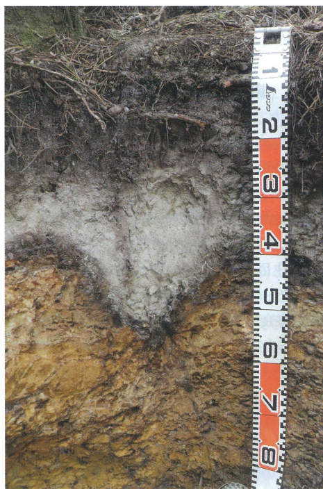
写真1. 第4段丘の土壌断面。漂白層の下にはっきりとしたBh層とBs層が観察された。
