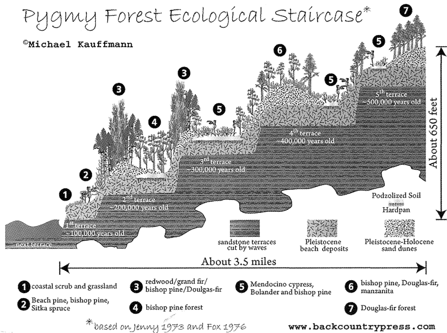
図2. 「生態系の階段 (Ecological Staircase)」の概念図 (Kauffmann, 2014)。
