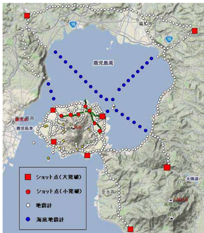
図2 観測点・ショット点全体配置
