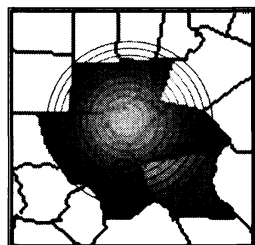
図 4.1 Circular スキャン
