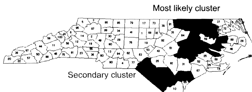
図 4.5 Echelon scan 法に基づく SIDS データのホットスポット
