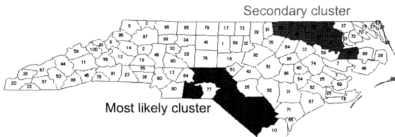
図 4.4 Flexible scan 法に基づく SIDS データのホットスポット
