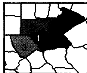
図 4.2 Flexible スキャン
