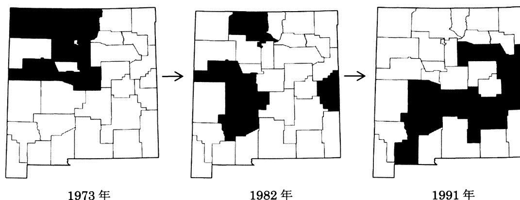
図 5.2 Echelon scan 法に基づく 3 年間分の悪性脳腫瘍死亡データの時空間ホットスポット
