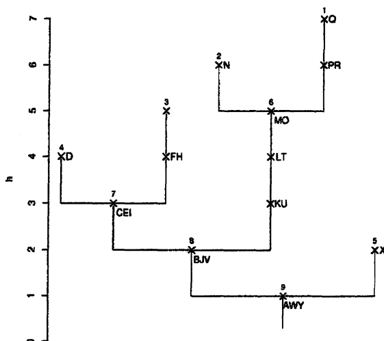
図 3.2 次元空間データのエシェロンデンドログラム
