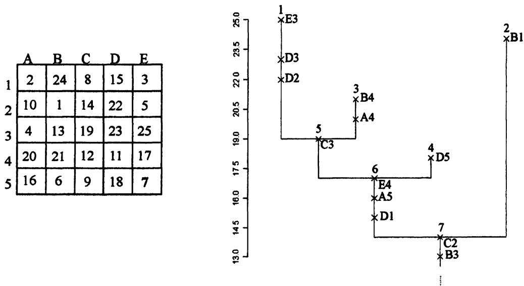
図 3.3 5×5 の空間データとそのエシェロンデンドログラム
