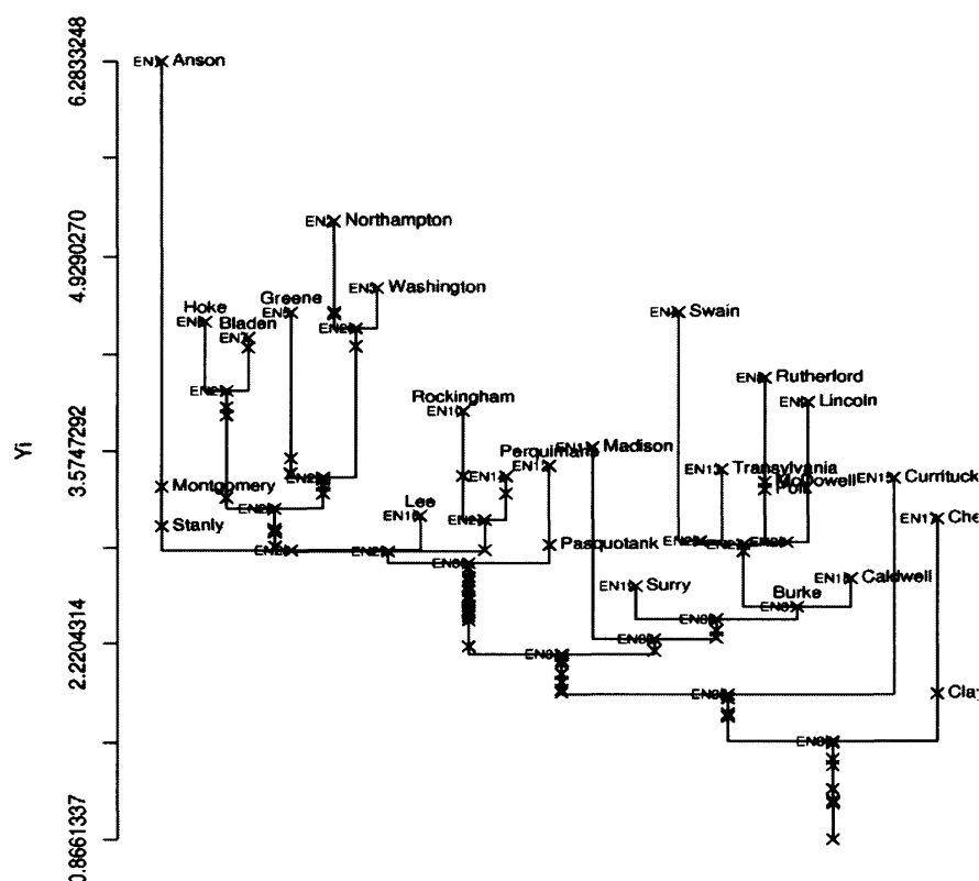
図 3.5 SIDS データの Echelon デンドログラム
