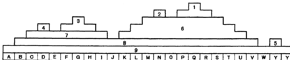
図 3.1 エシェロン解析における同じ位相領域への分割
