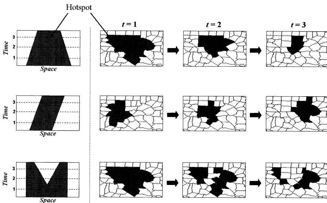
図 5.1 時空間ホットスポットの例
