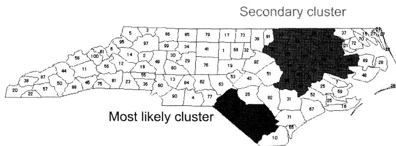
図 4.3 Circular scan 法に基づく SIDS データのホットスポット
