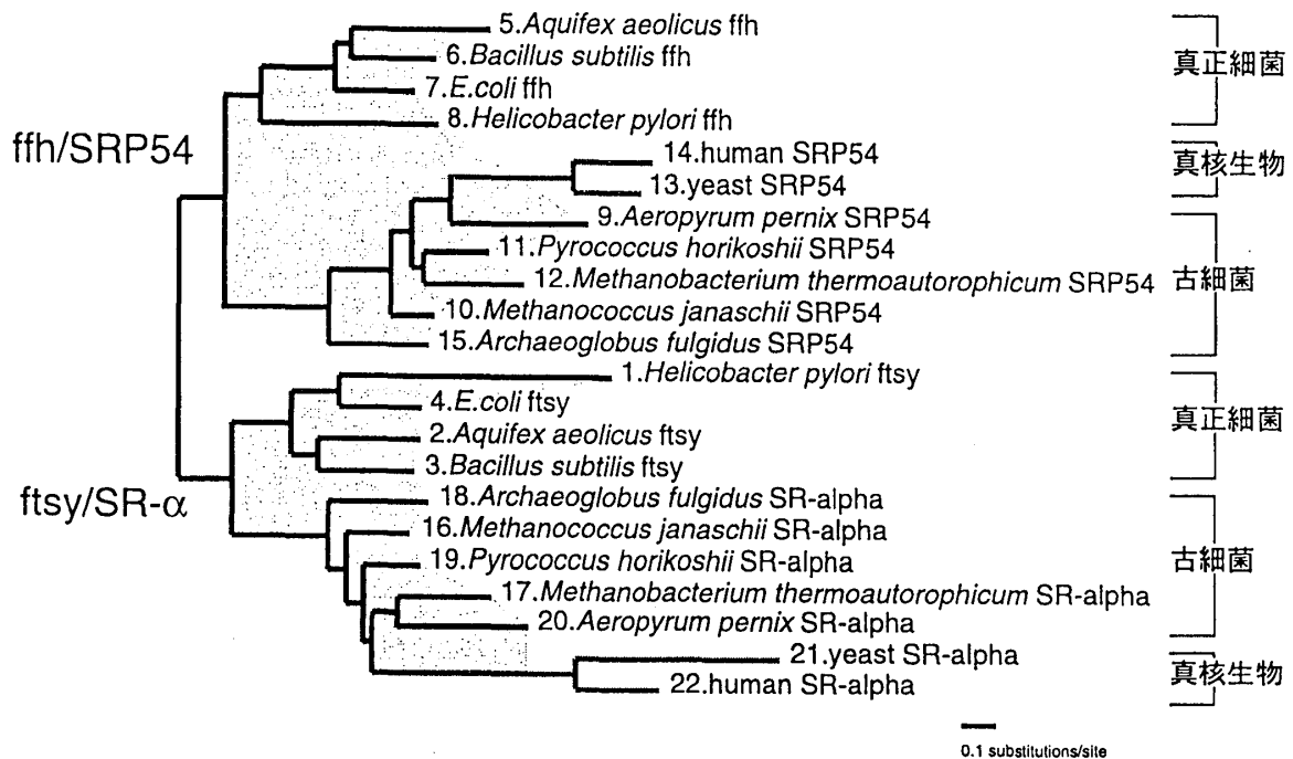
図 3: パラログな遺伝子を用いたルートの特定
