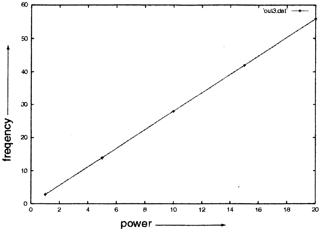
図9. Ⅲのパラメータ領域におけるリミットサイクル振動の周波数とビーム強度 P の関係。
