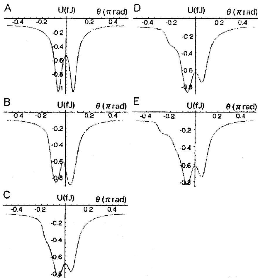
図6. 1接点剛体棒モデルに対するポテンシャルエネルギーの計算結果。それぞれは異なる \phi の値に対応し、A: \phi=0\pi\text{rad} 、B: \phi=0.1\pi\text{rad} 、C: \phi=0.2\pi\text{rad} 、D: \phi=0.3\pi\text{rad} 、E: \phi=0.4\pi\text{rad} の場合を示す。
