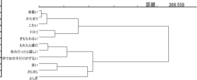
図1. Sのデンドログラム
