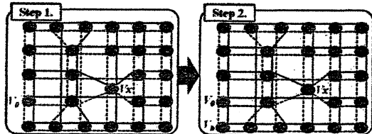
図 14: DeleteMultipleRows の Step1~2.
