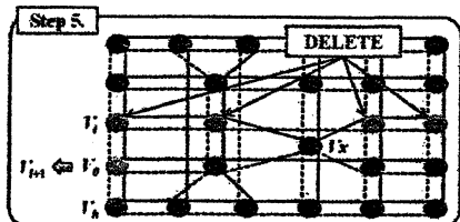
図 16: DeleteMultipleRows の Step5.
