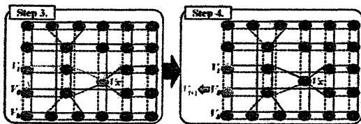
図 15: DeleteMultipleRows の Step3~4.
