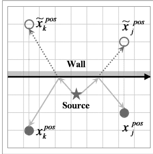
図 3: 観測点とその鏡像点, 信号源, 壁の位置関係.
