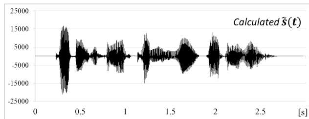
図 7: 分離された信号源 \tilde{s}(t)/a_{11} の時刻歴.
