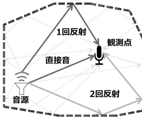
図 1: 凸多角形内部で信号が伝わる様子。
