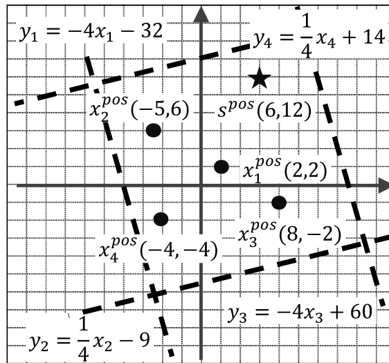
図 4: 信号源，観測点，壁の設定図．
