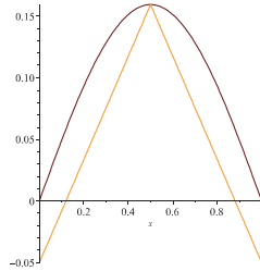
図 1: 障害物が \psi(1/2) \approx 0.16 の時の (M) の解.
